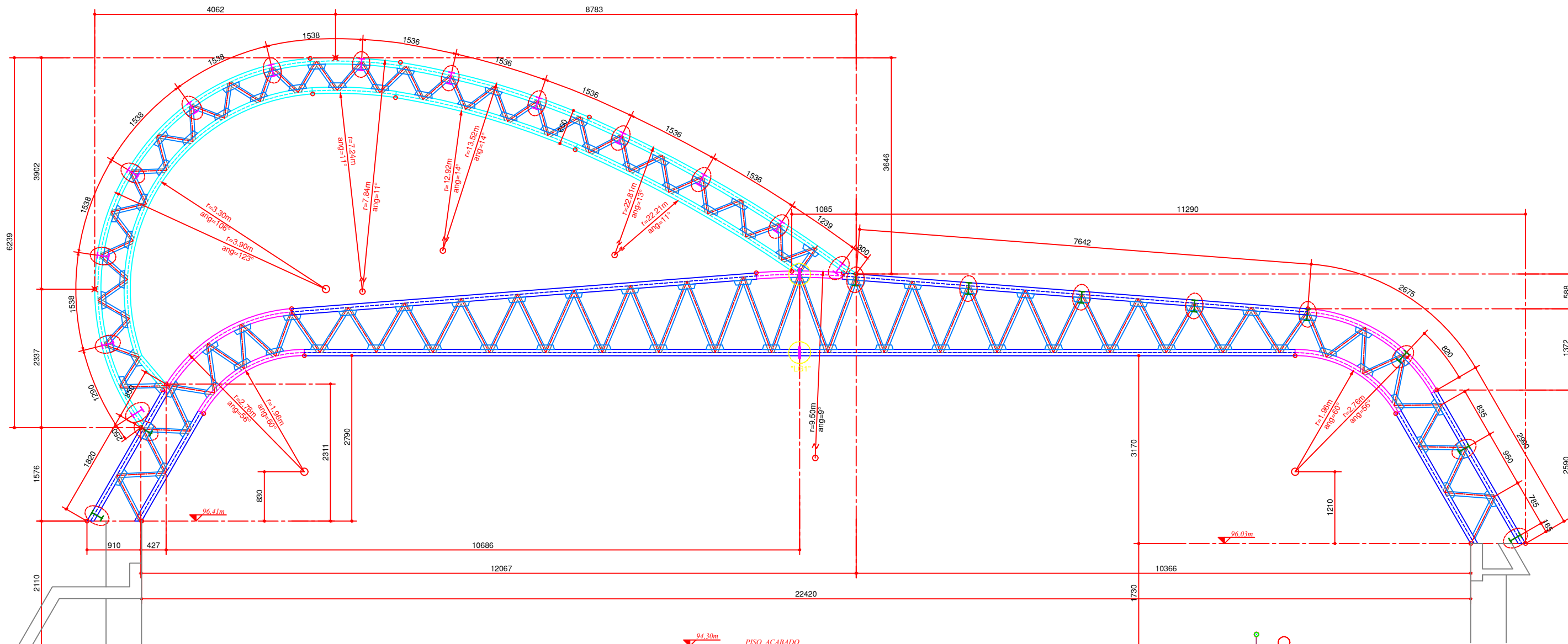
DETALHE PÓRTICO - EIXO R6
