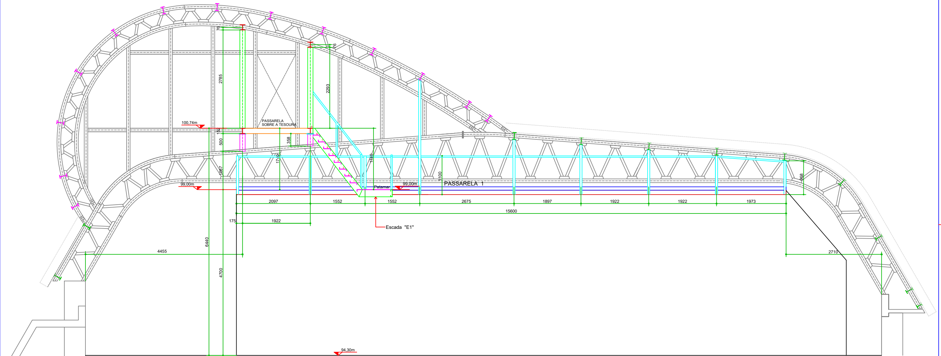
CORTE - C1 (EIXO E1A)
