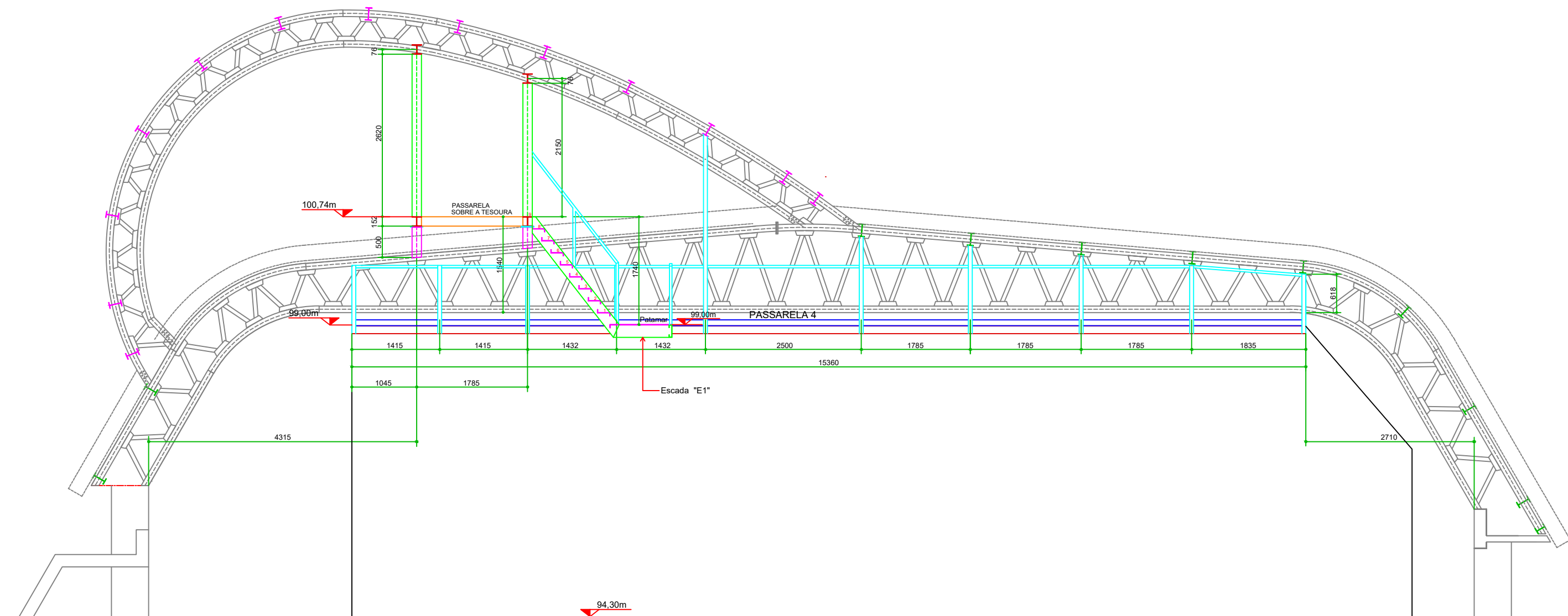
CORTE - C4 (EIXO R4)
