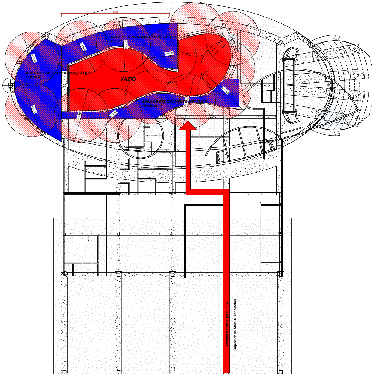
1 PLANTA DE ESCORAMENTO 1:100
