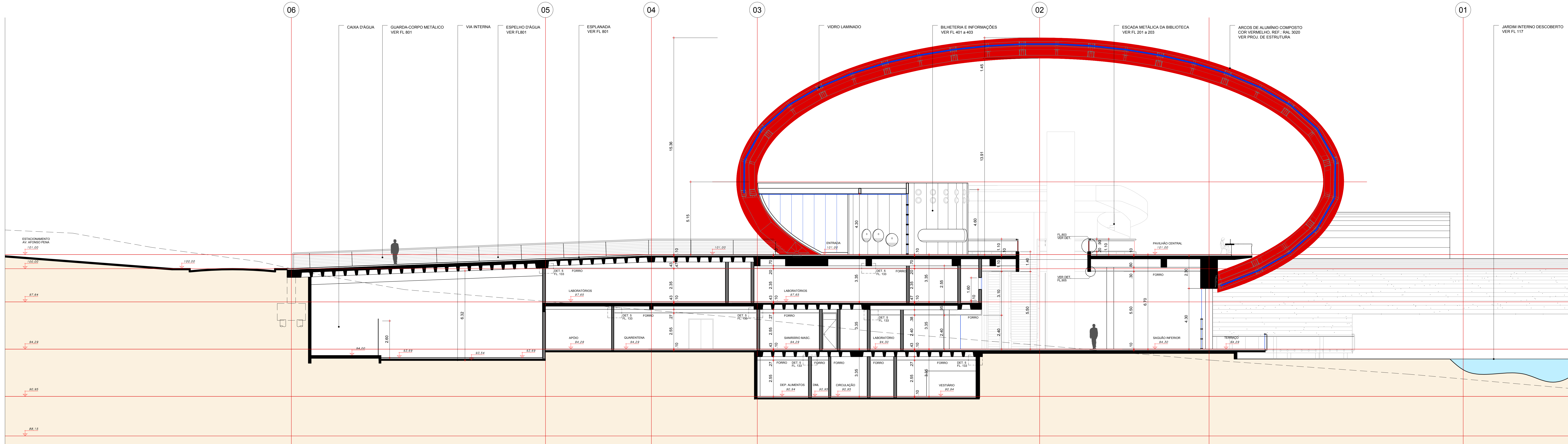
CORTE A ESCALA 1:100
