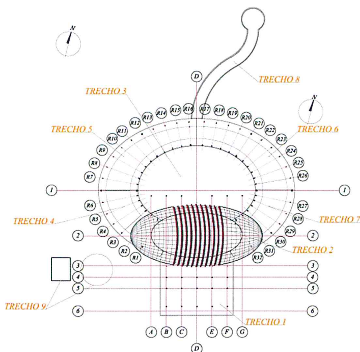
PLANTA CHAVE ESC. 1:500
