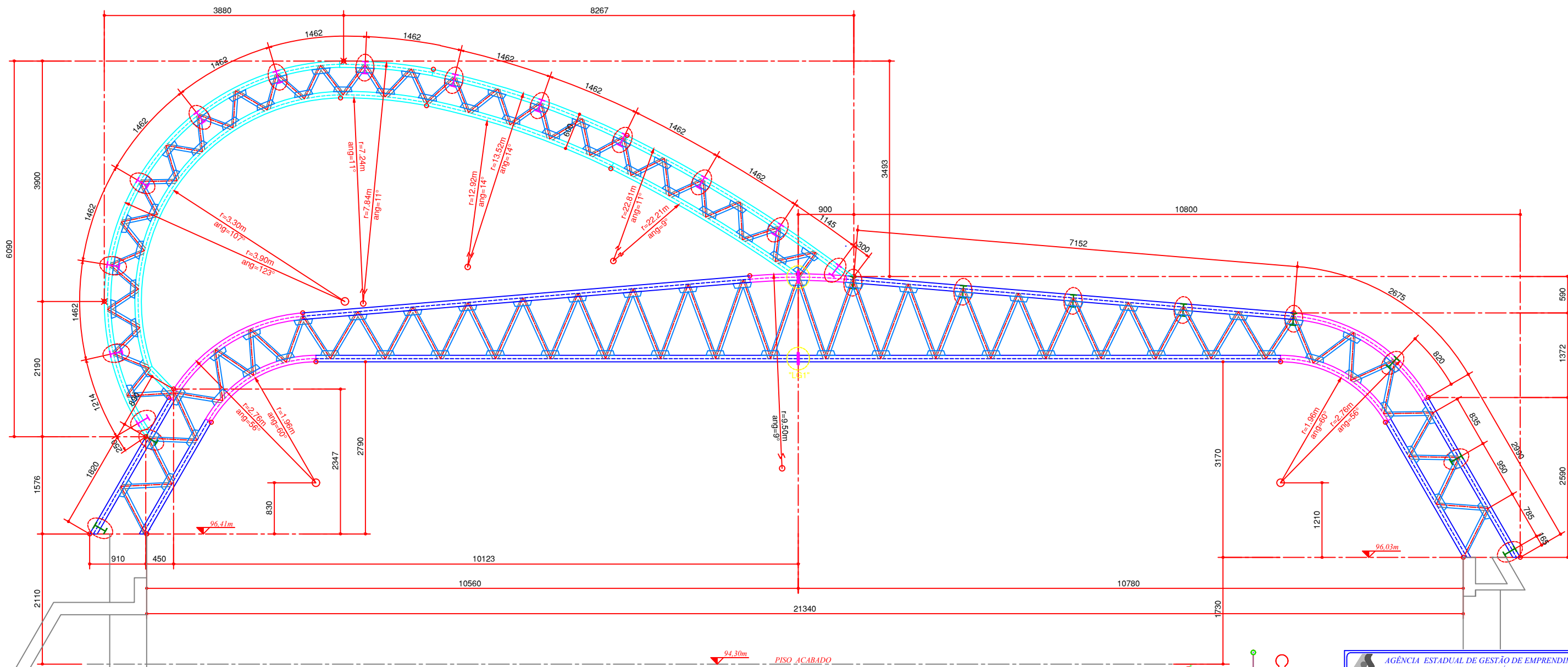
DETALHE PÓRTICO - EIXO R4
