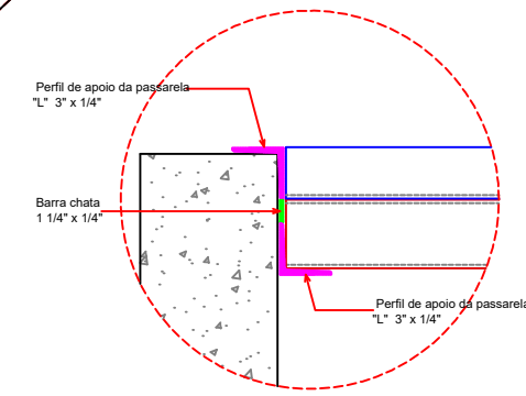
DETALHE APOIO "AP1"
