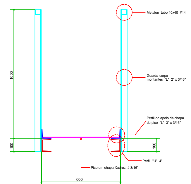
CORTE TRANSVERSAL NAS PASSARELAS Escala: 1/7,5
