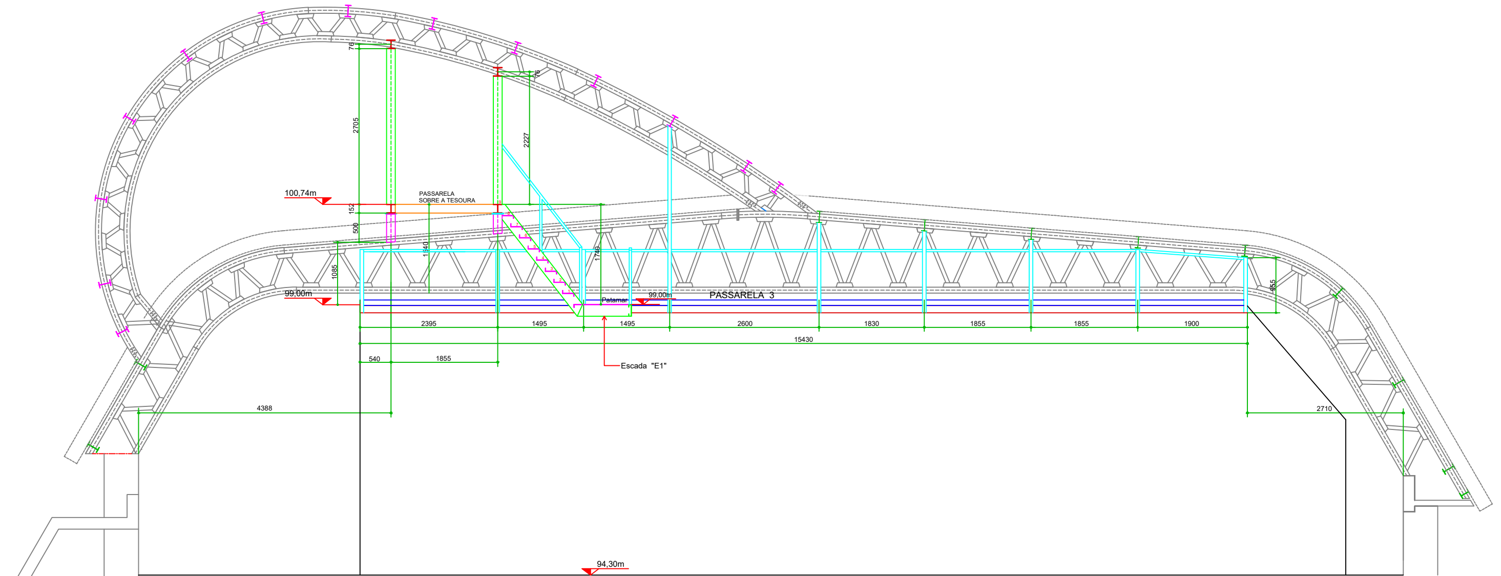
CORTE - C3 (EIXO R5)
