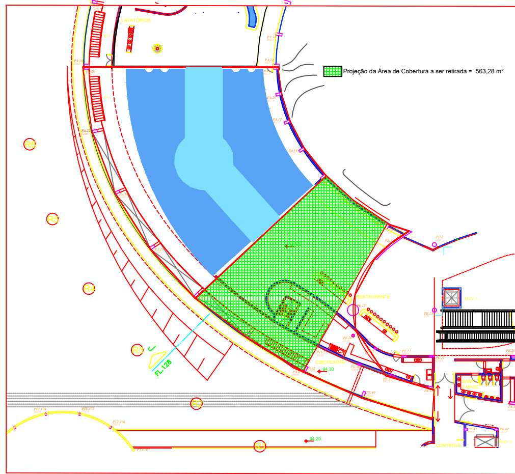
PROJEÇÃO COBERTURA 02
