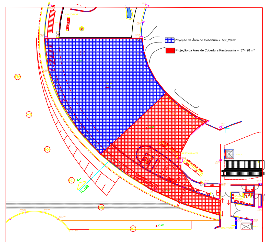
PROJEÇÃO COBERTURA 01
