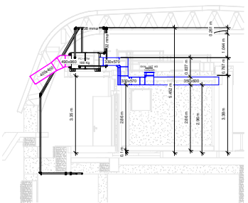
4 Corte Sanitário 94.30 Trecho 5 1:50
