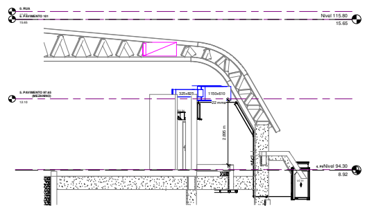
2 Corte 02 1:150
