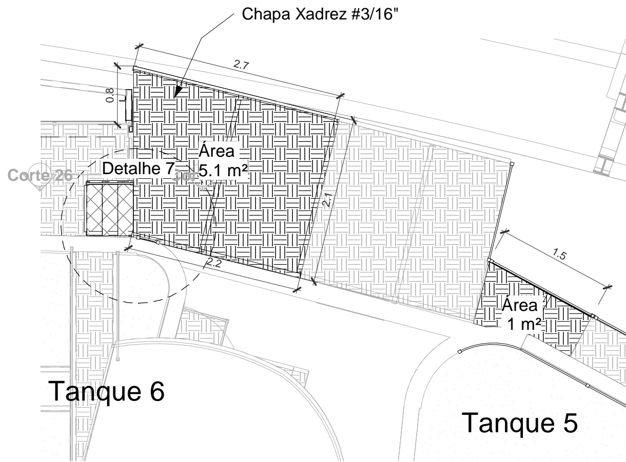
Detalhamento 1.0
