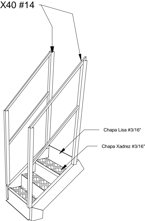
Detalhe Escada metálica
