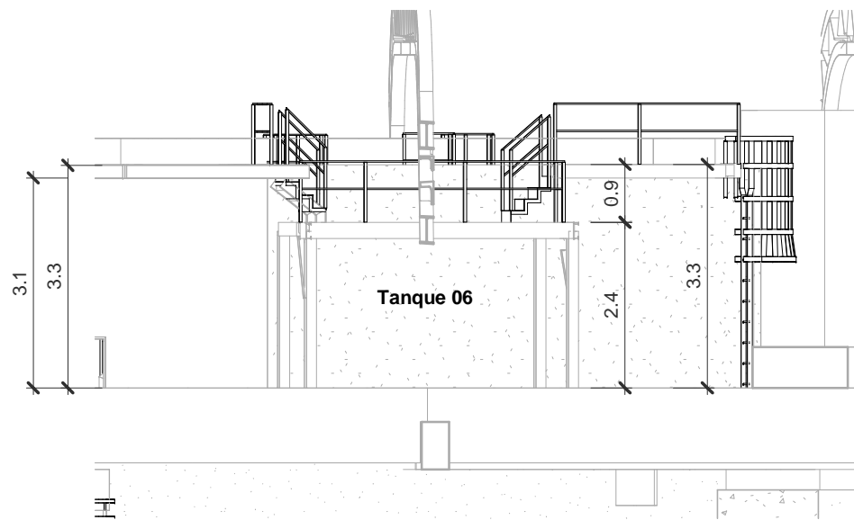
Corte 3
