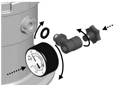
Montagem manômetro (válvula top)
