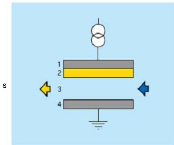
Fig. 1: Ozone generation 1 : High voltage electrode 2 : Dielectric 3 : Discharge gap 4 : Earth electrode
