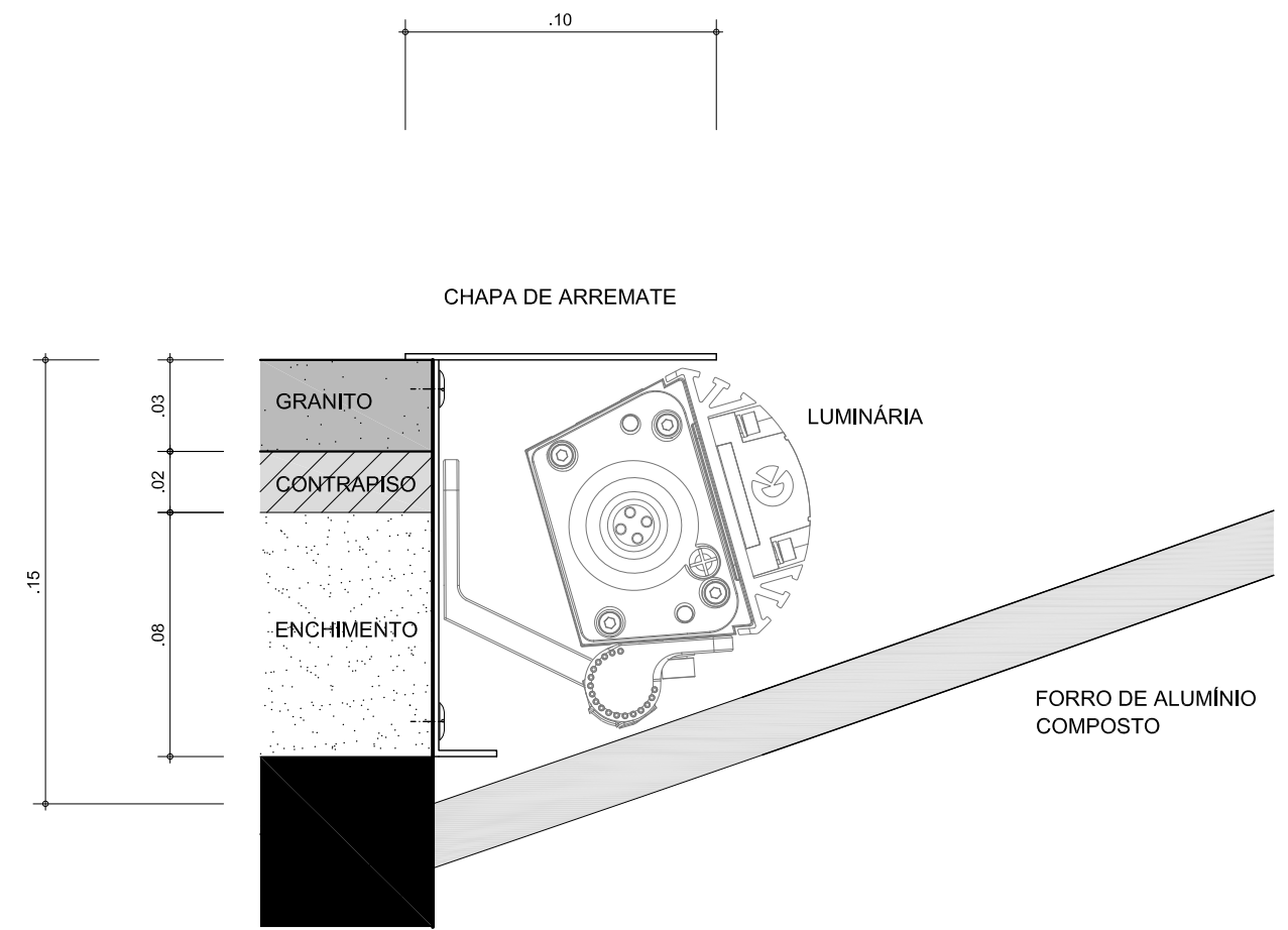
SEÇÃO - ENCONTRO PISO COM O FORRO ESC.: 1:2,5 ( VIGA )
