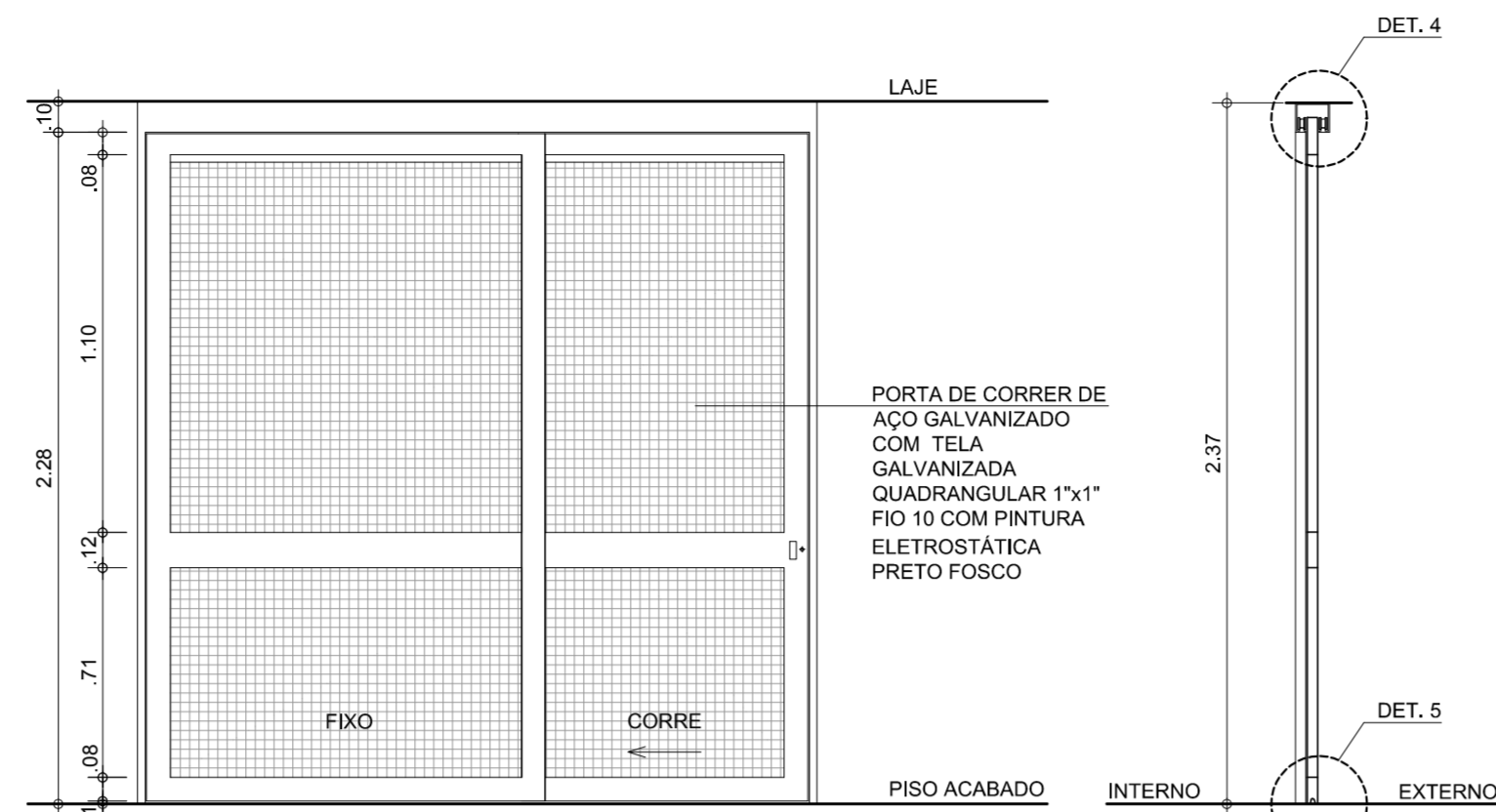
ELEVAÇÃO - PF4 ESC. 1:25
