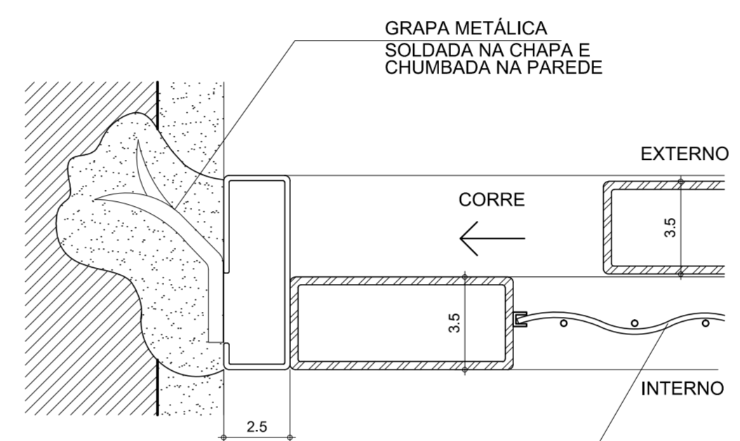
DET. 3 CORTE ESC. 1:2
