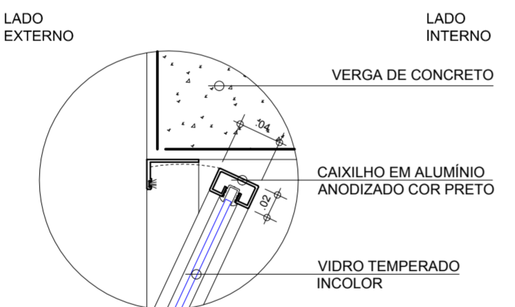
DET. 6 ESC. 1:5
