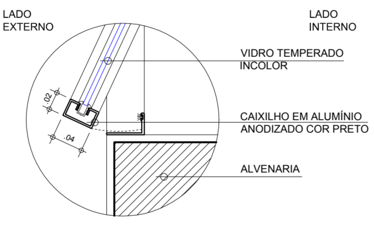
DET. 7 ESC. 1:5
