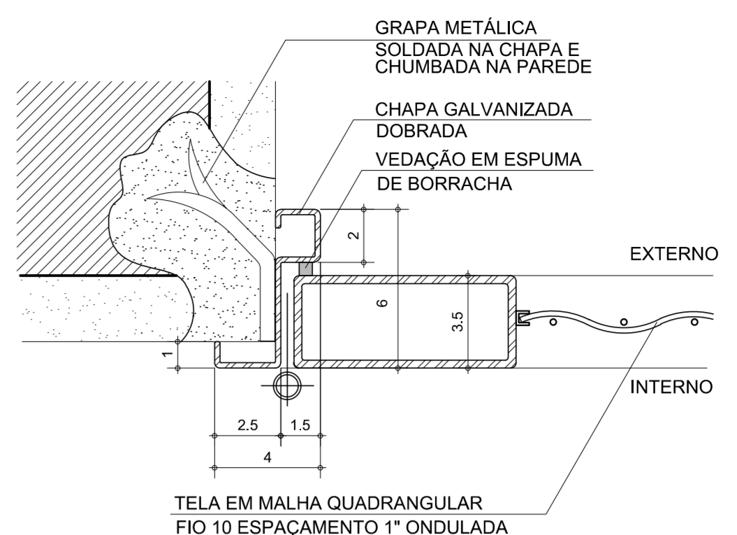
DET. 2 PLANTA ESC. 1:2
