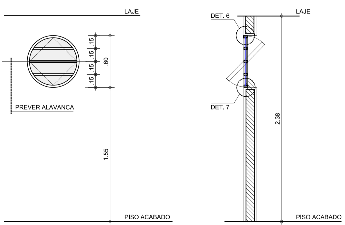
ELEVAÇÃO 1 - CF 21 ESC. 1:25
