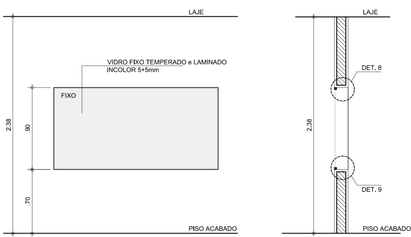
ELEVAÇÃO - VT14 ESC. 1:25
