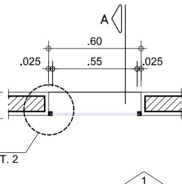
PLANTA - CF 21 ESC. 1:25
