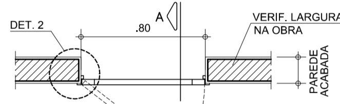
PLANTA - PF3 ESC. 1:25
