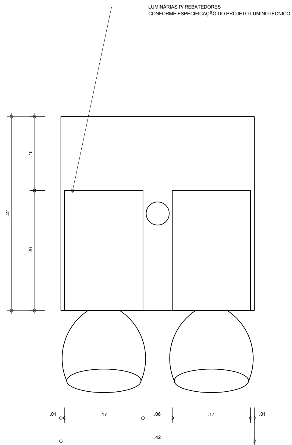
PLANTA NIVEL 1
