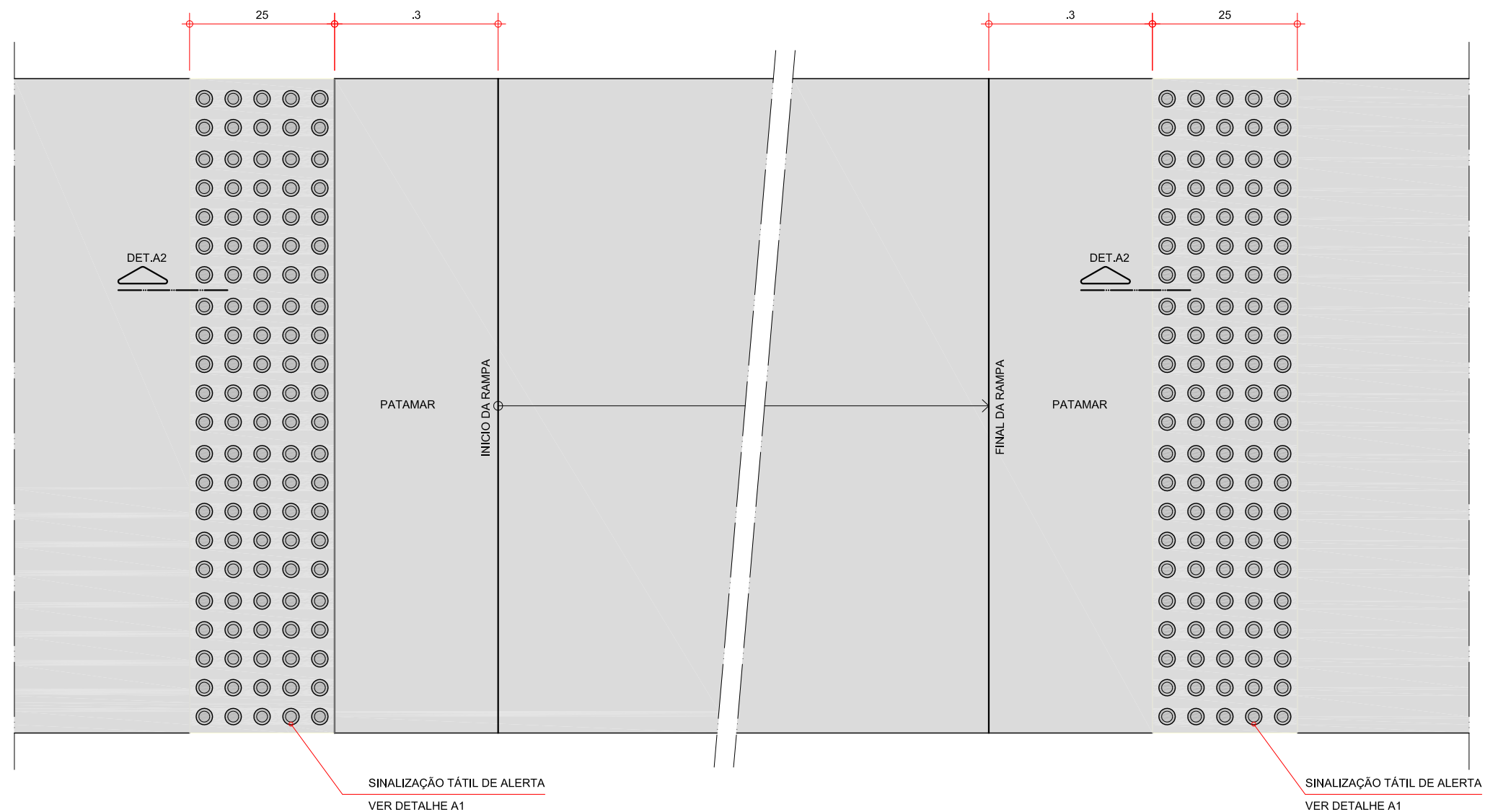
DETALHE SINALIZAÇÃO TÁTIL NA RAMP ESCALA 1:10
