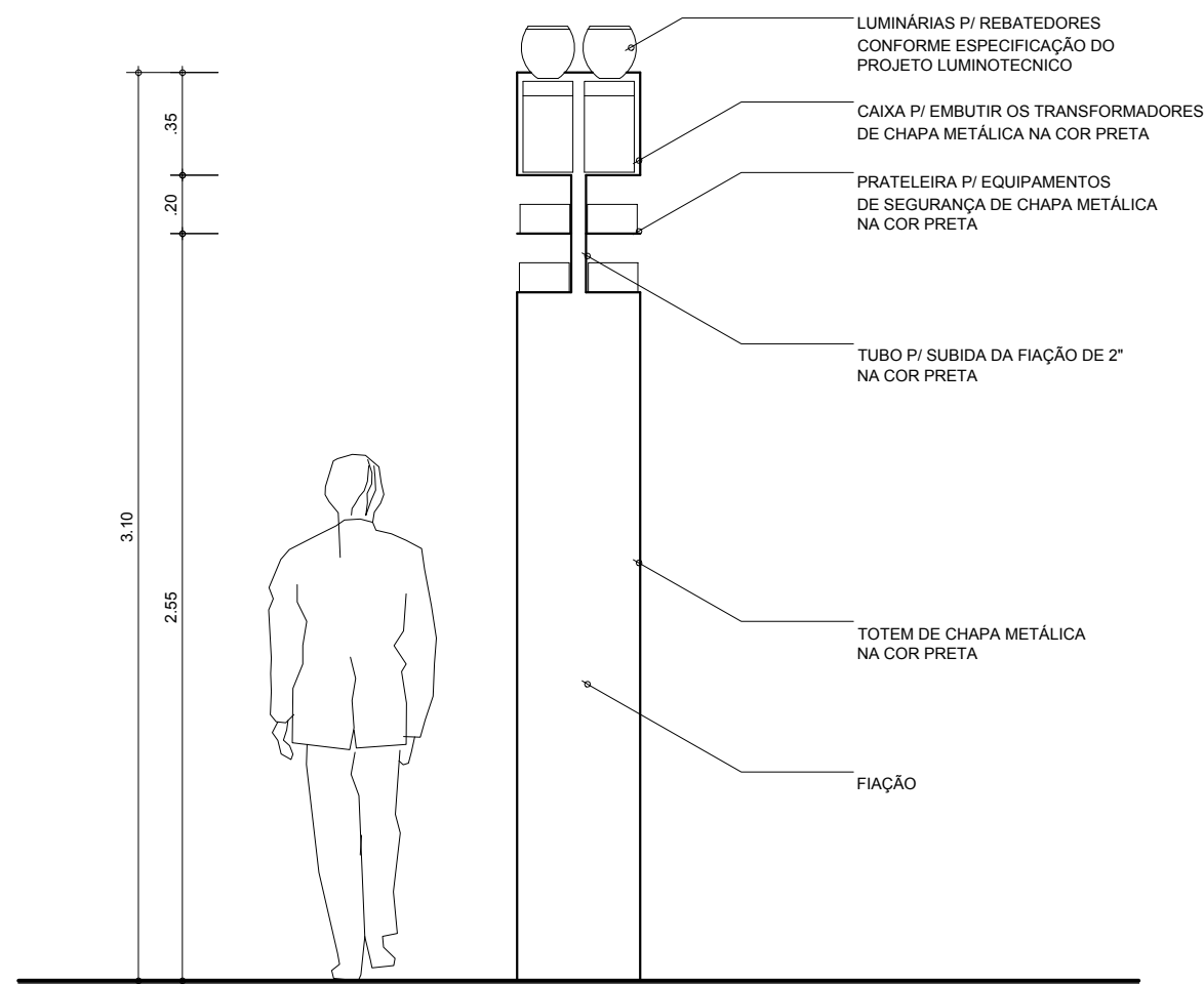
SEÇÃO ESCALA 1:20
