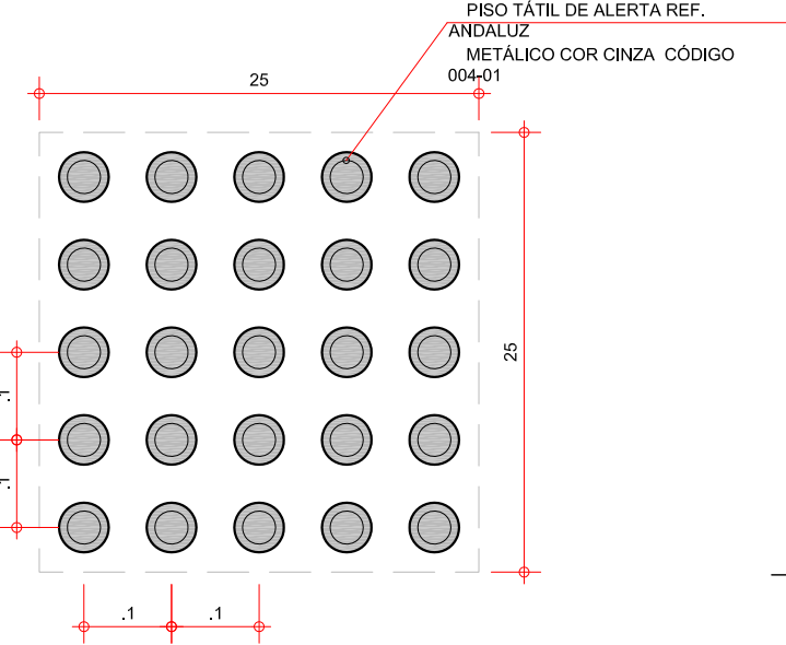
DETALHE A1
