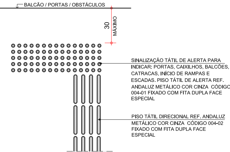
DETALHE S1 SINALIZAÇÃO TÁTIL DE ALERTA E DIRECIONAL ESCALA 1:20
