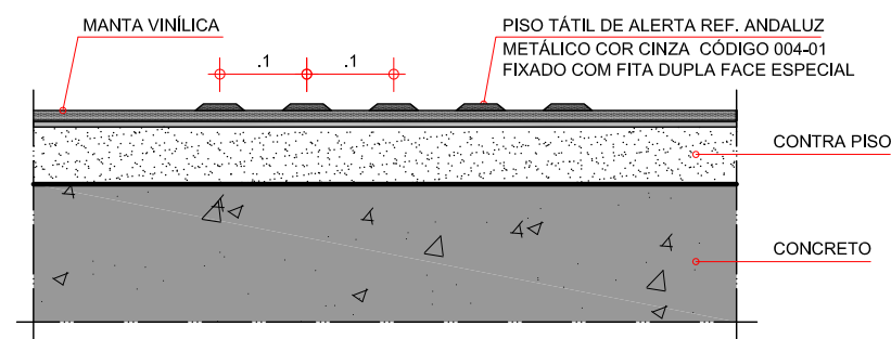
DETALHE A2 ESCALA 1:5
