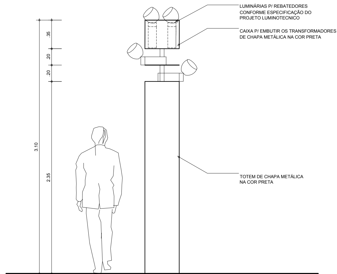
ELEVAÇÃO ESCALA 1:20
