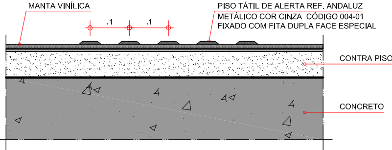
DETALHE A2
