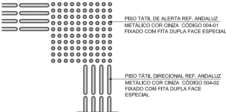
DETALHE S2 SINALIZAÇÃO TÁTIL DE ALERTA E DIRECIONAL ESCALA 1:20
