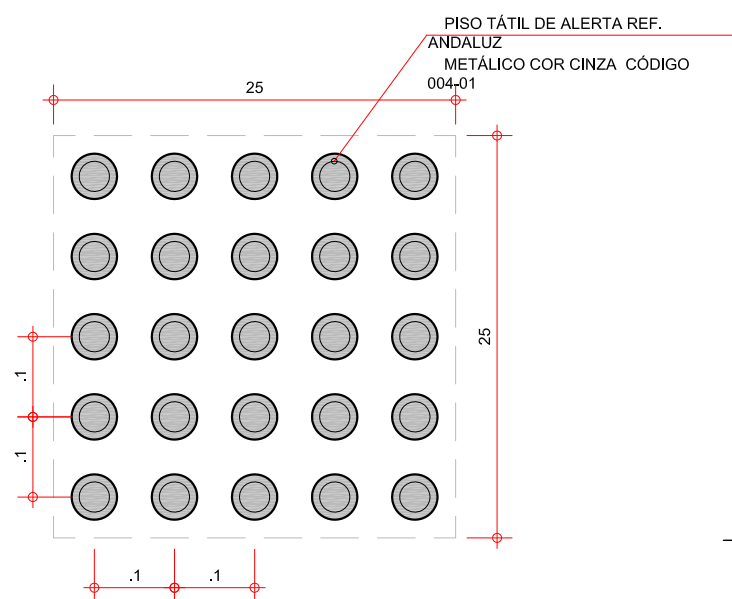
DETALHE A1 ESCALA 1:5
