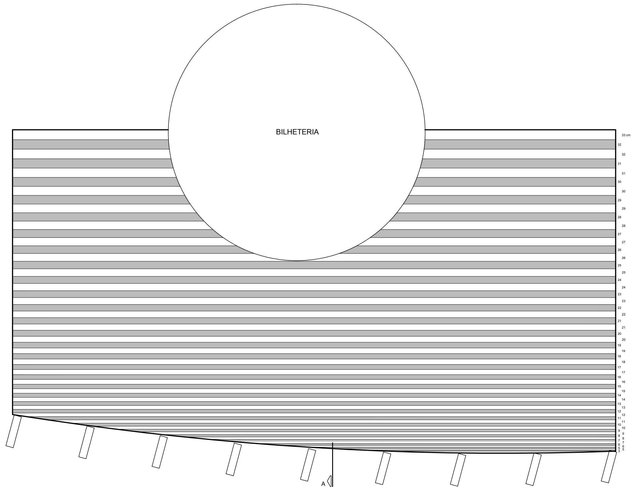
CAIXILHO CF1 PLANTA DE COBERTURA ESC. 1:75
