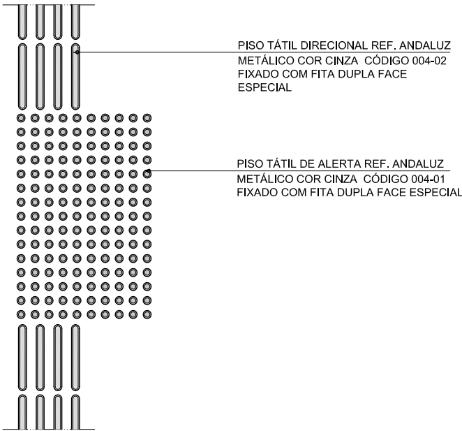
DETALHE S3 SINALIZAÇÃO TÁTIL DE ALERTA E DIRECIONAL ESCALA 1:20
