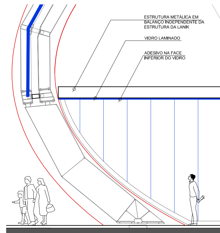
SEÇÃO A ESC. 1:75
