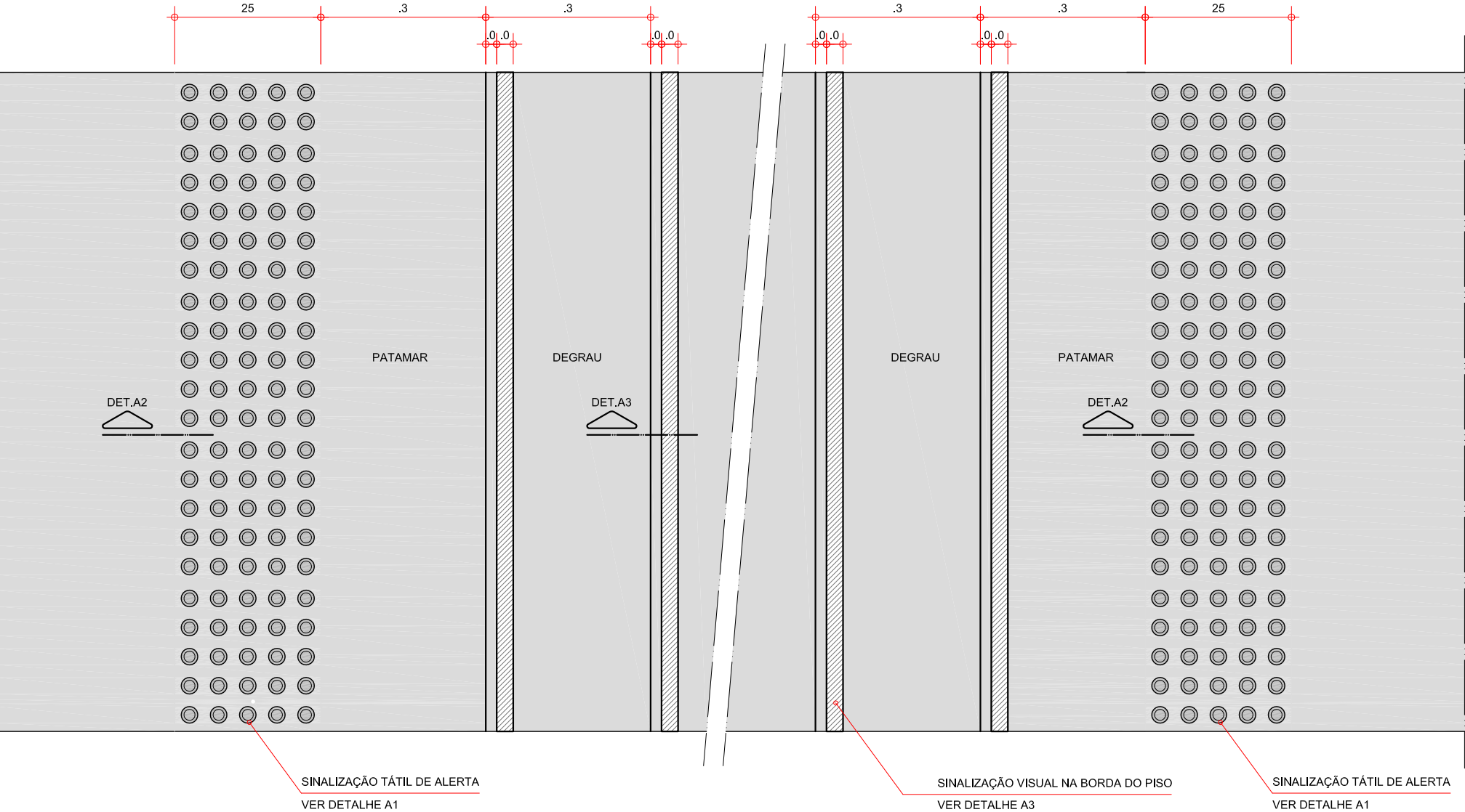
DETALHE SINALIZAÇÃO TÁTIL E VISUAL DOS DEGRAUS DA ESCADA
