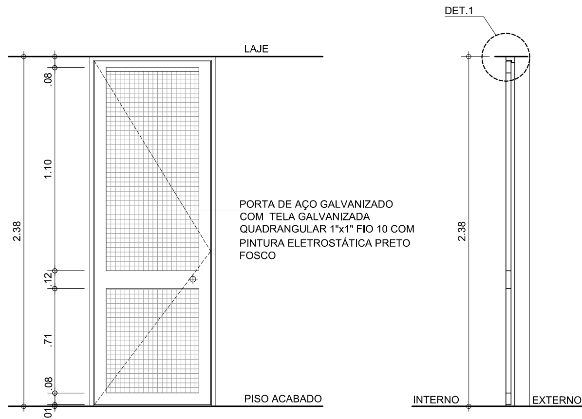
ELEVÇÃO - PF3
