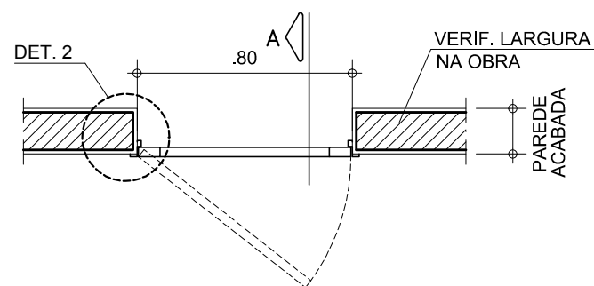
PLANTA - PF3
