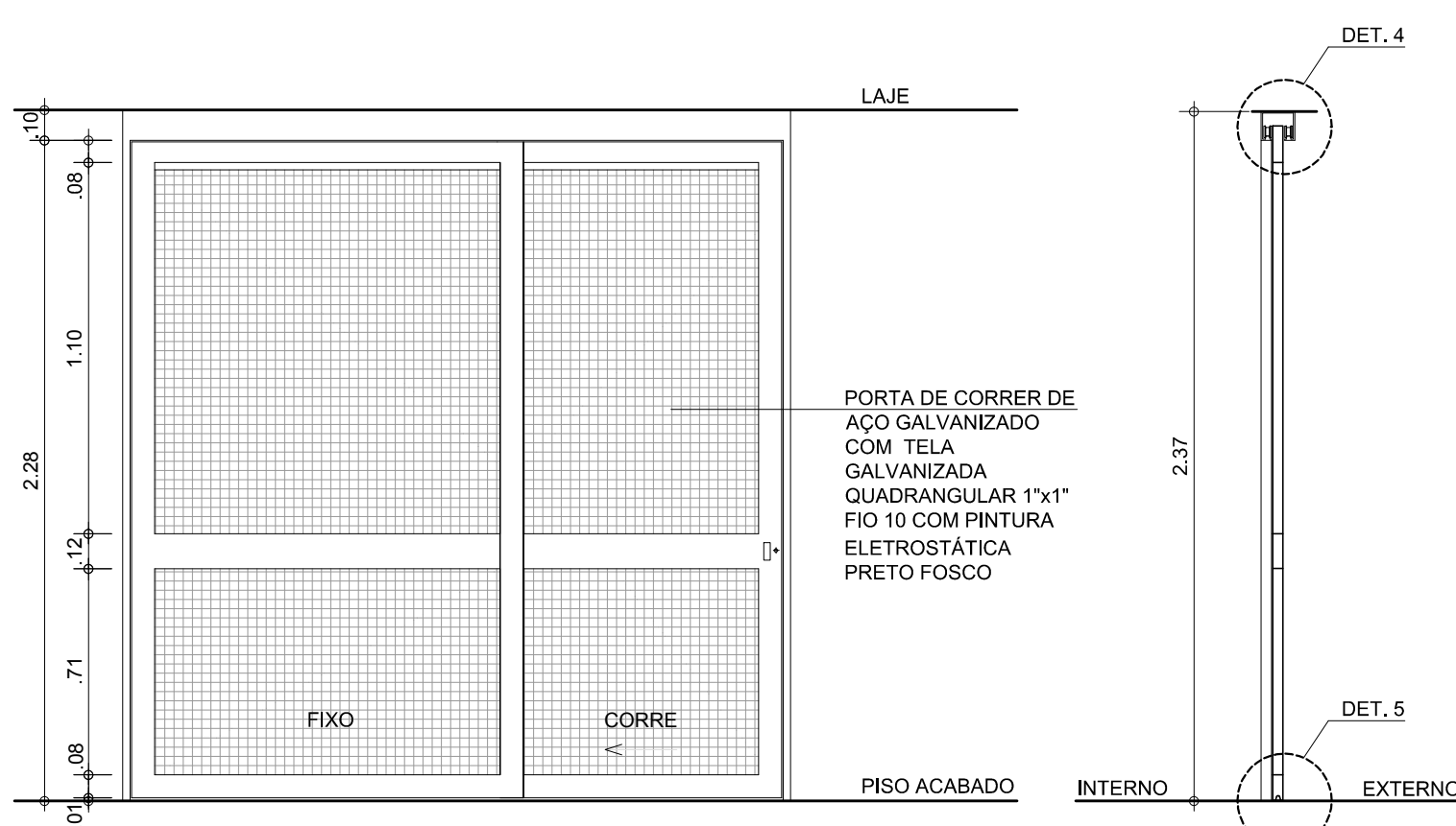
ELEVÇÃO - PF4
