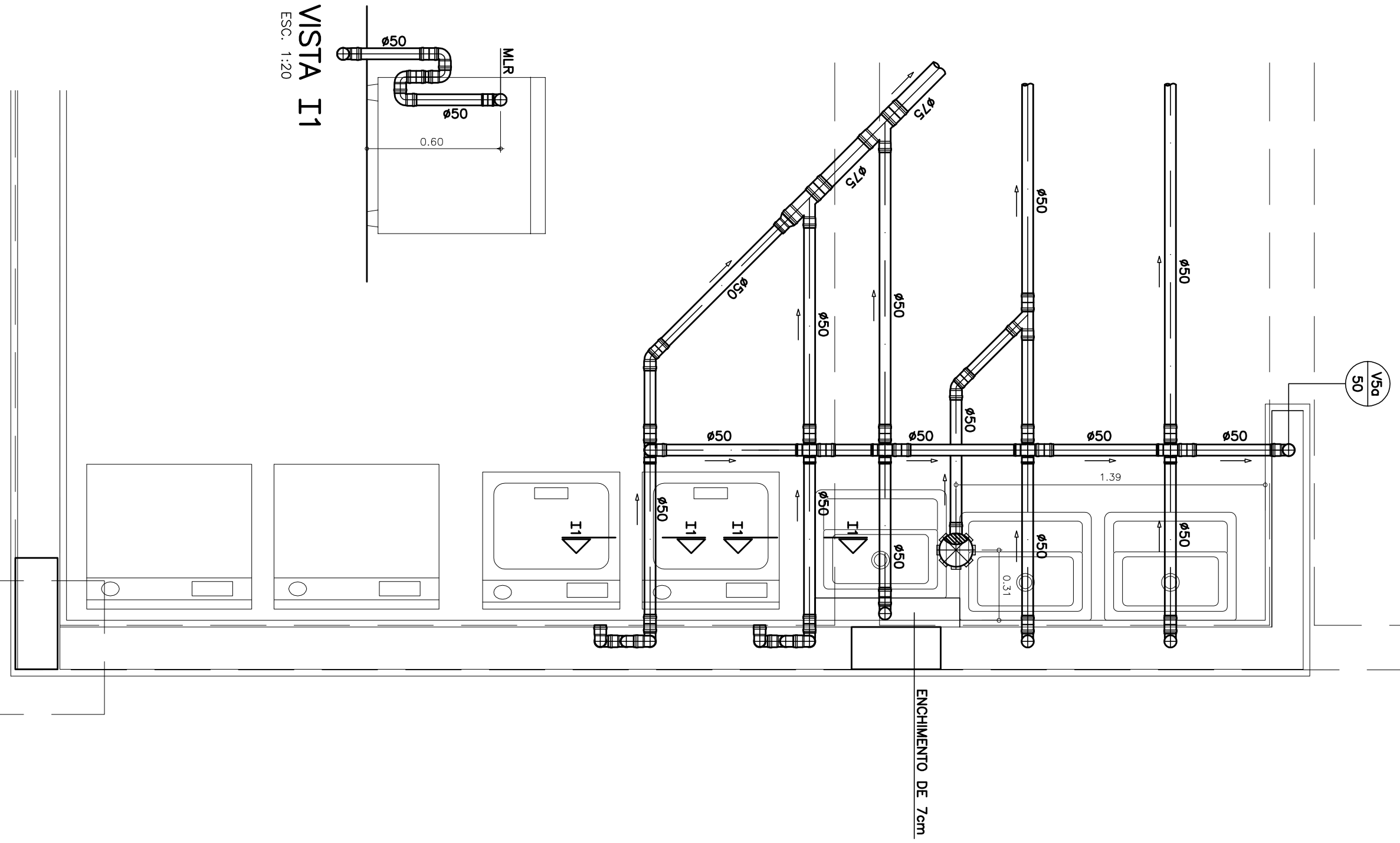
DETALHE I1 - NÍVEL 94,30 ESC. 1:20
