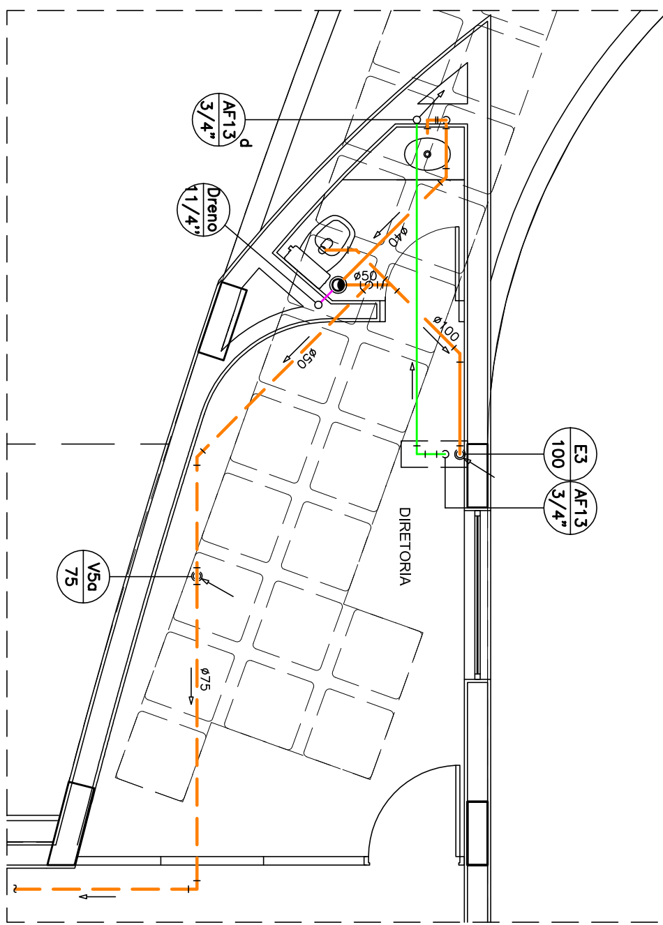
DETALHE © – NÍVEL 97,65
