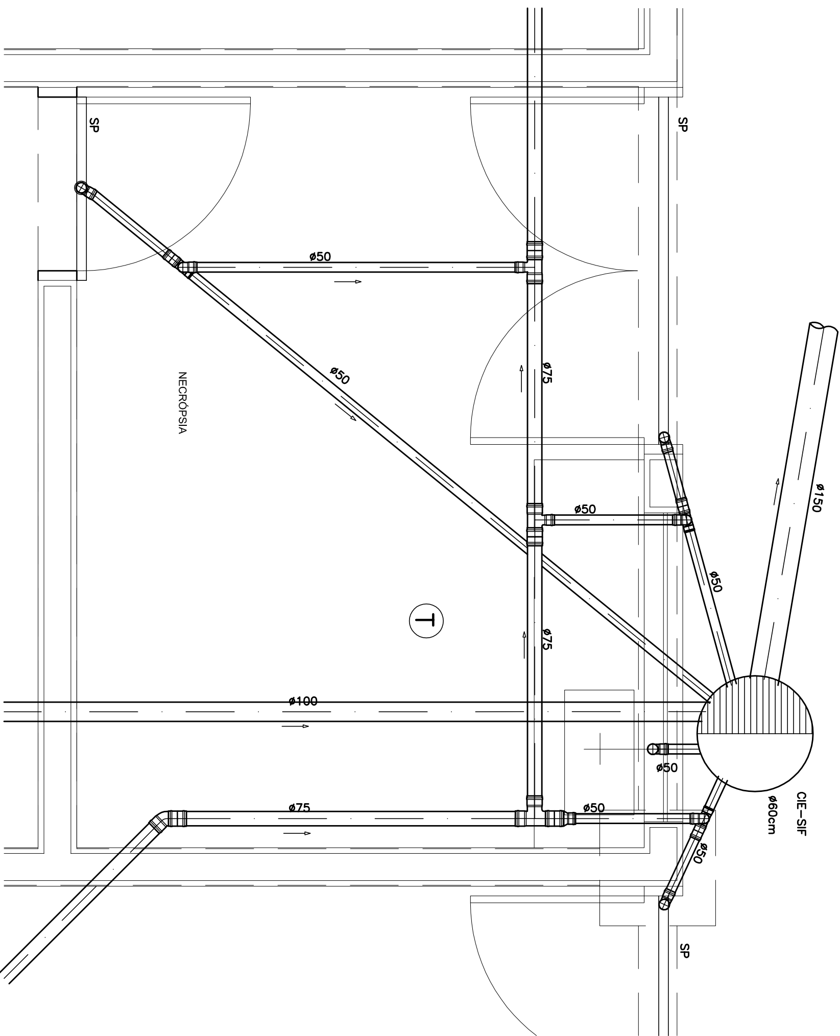
DETALHE T – NIVEL 90,95
