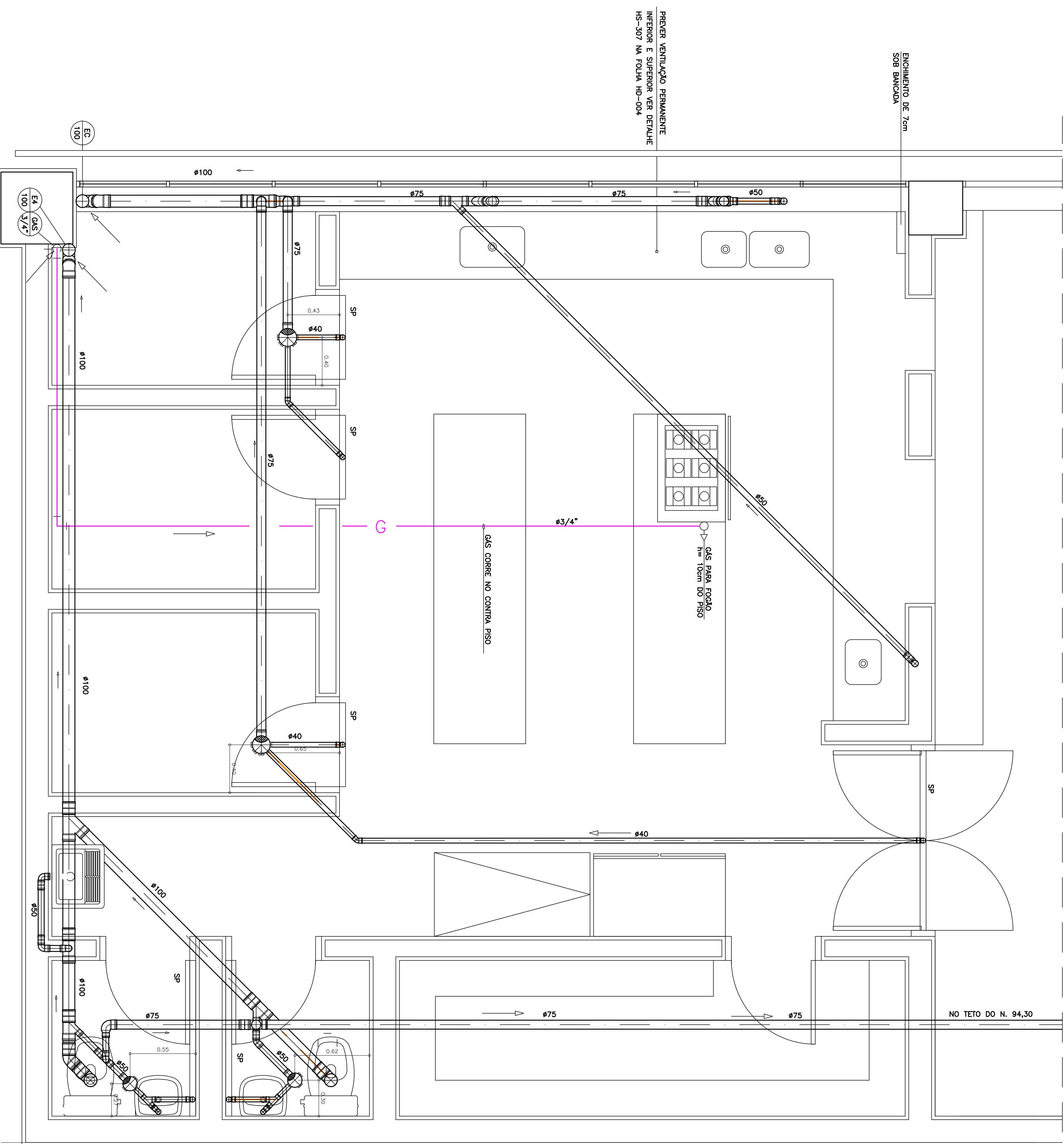
DETALHE D - NIVEL 97.65
