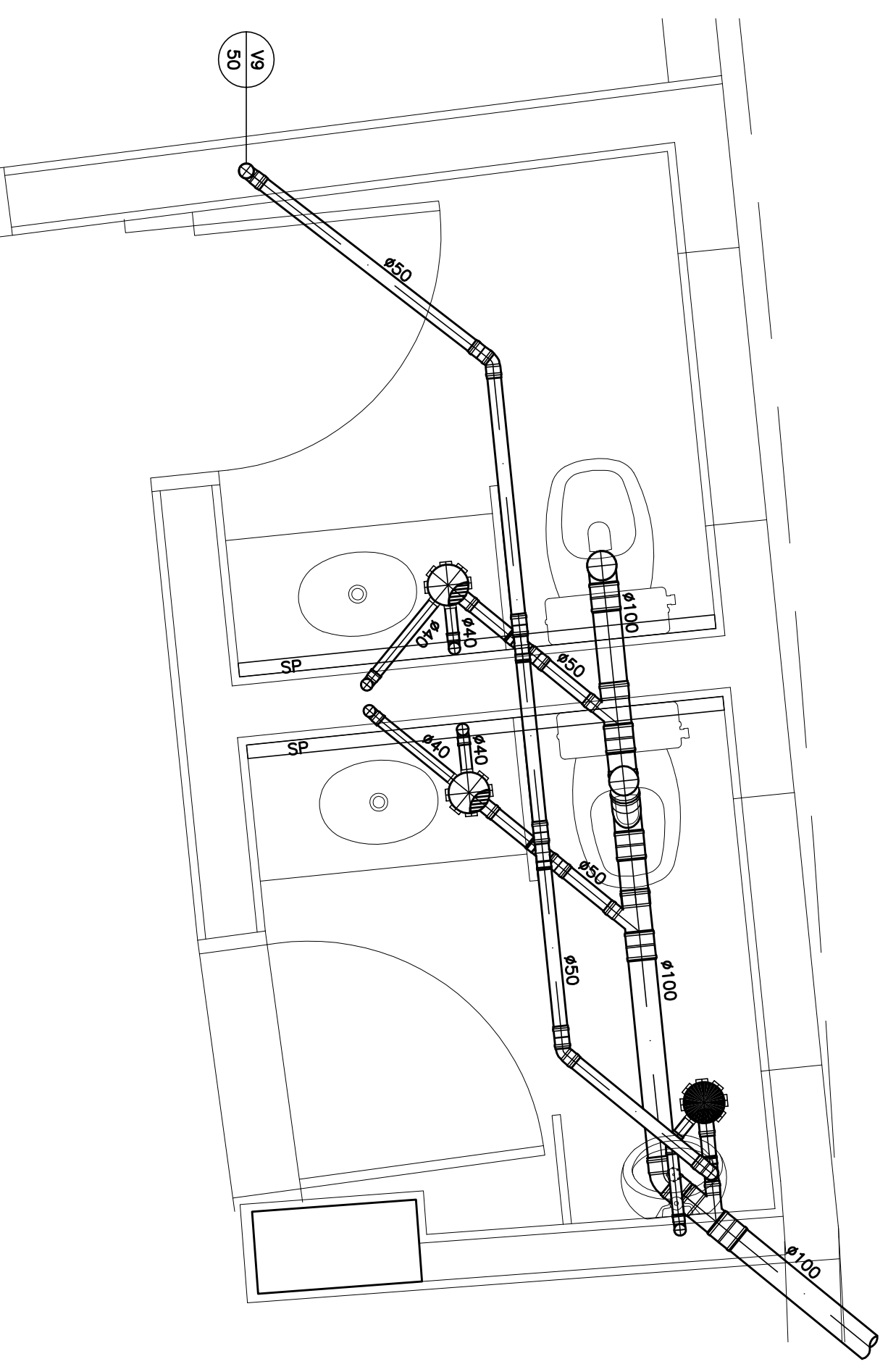
DETALHE L – NÍVEL 85,35
