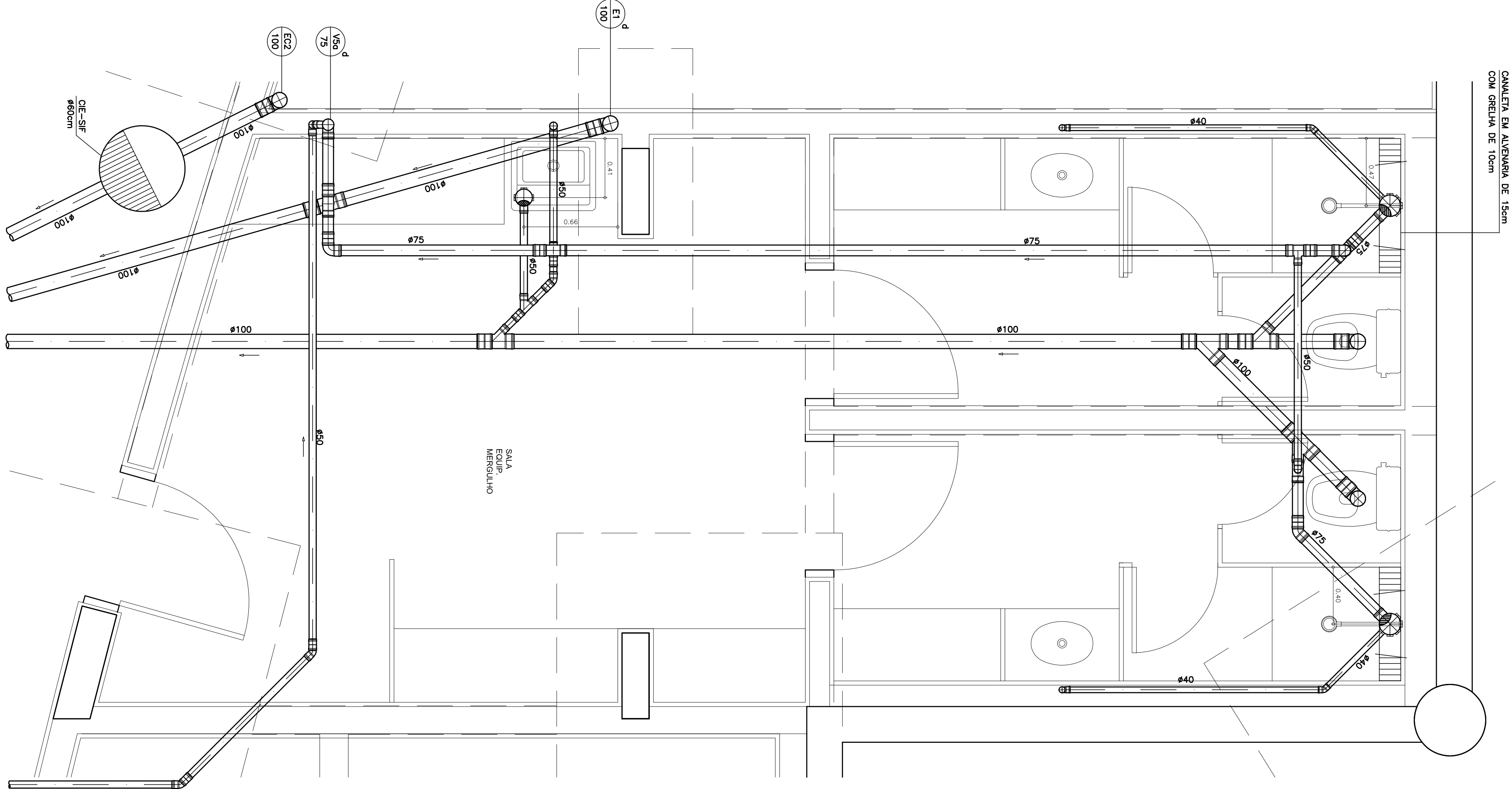
DETALHE M – NIVEL 90,95
