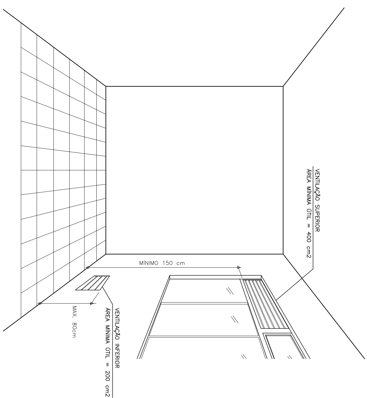
COZINHA VENTILAÇÃO PERMANENTE SUPERIOR E INFERIOR HS-307 S/ESCALA
