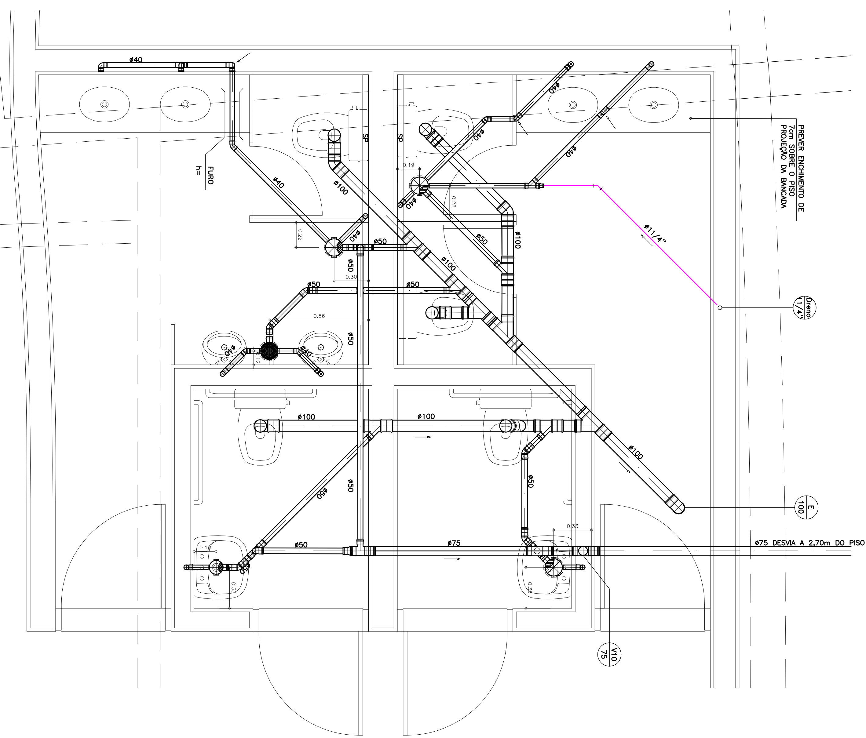
DETALHE J – NIVEL 85,35
