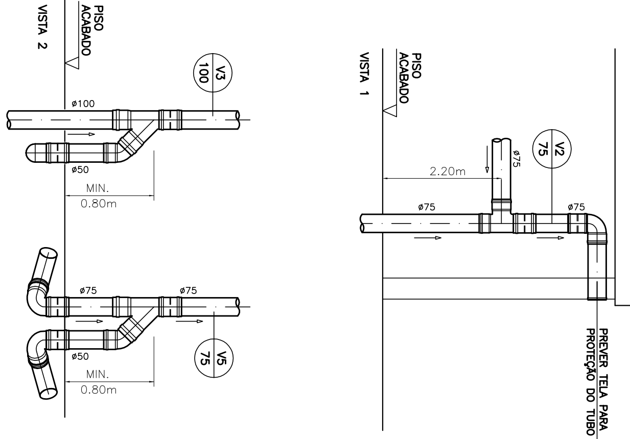
DETALHE VENTILAÇÃO INTERLIGAÇÃO A COLUMNA
