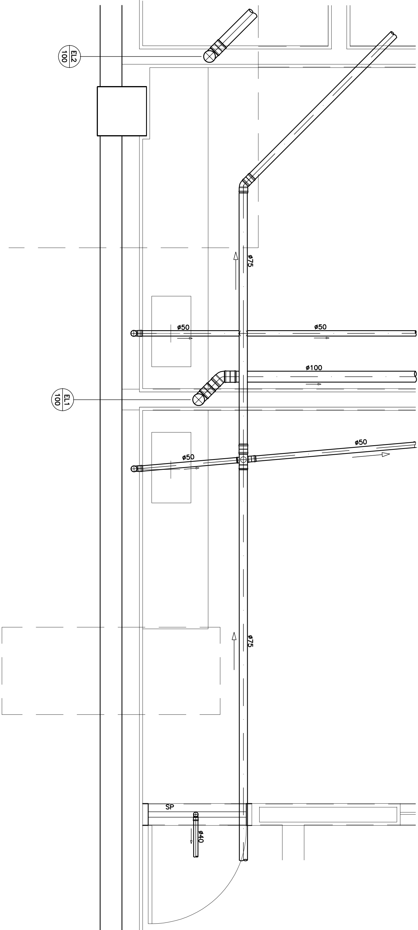
DETALHE S – NIVEL 90,95
