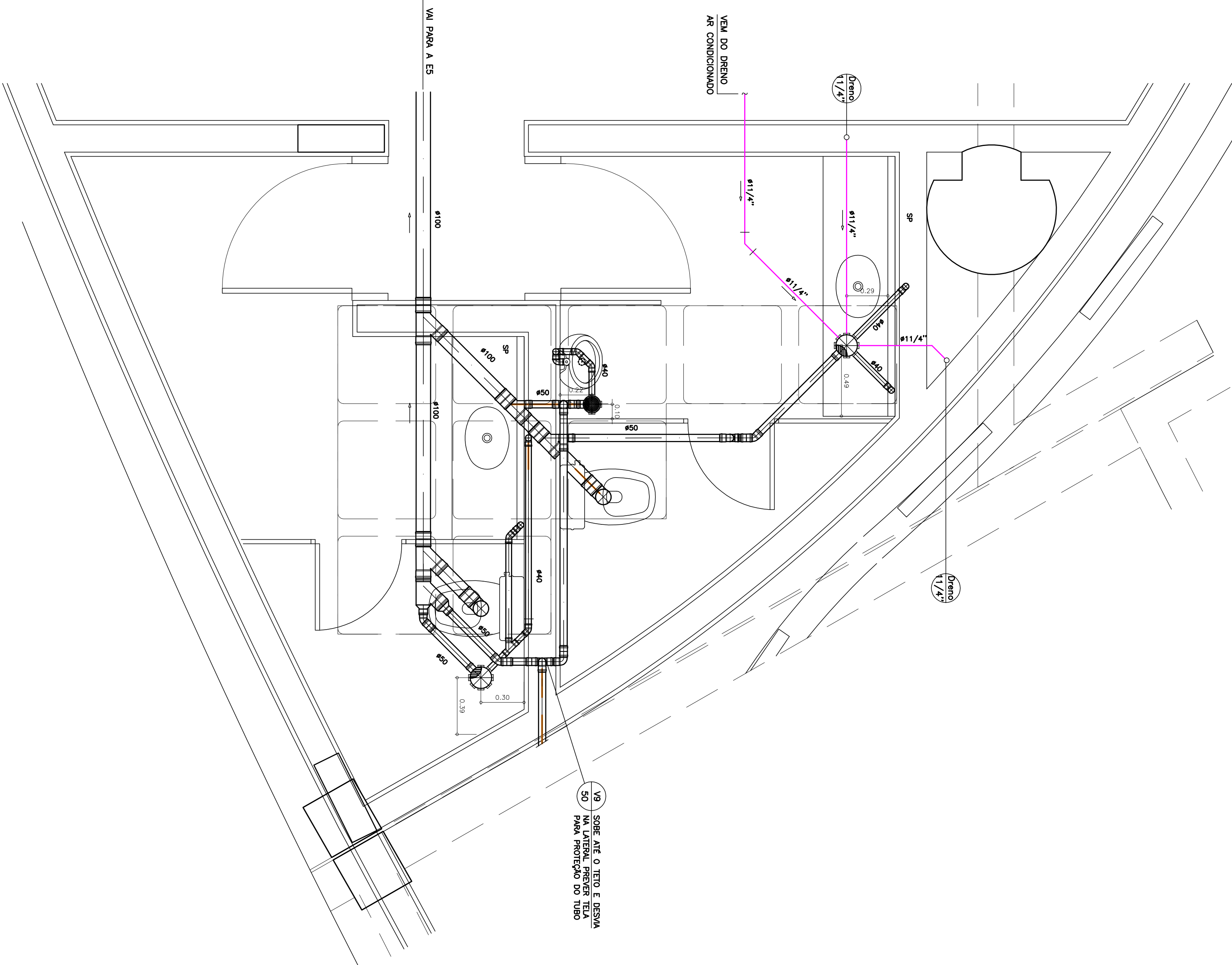
DETALHE E - NIVEL 94.30
