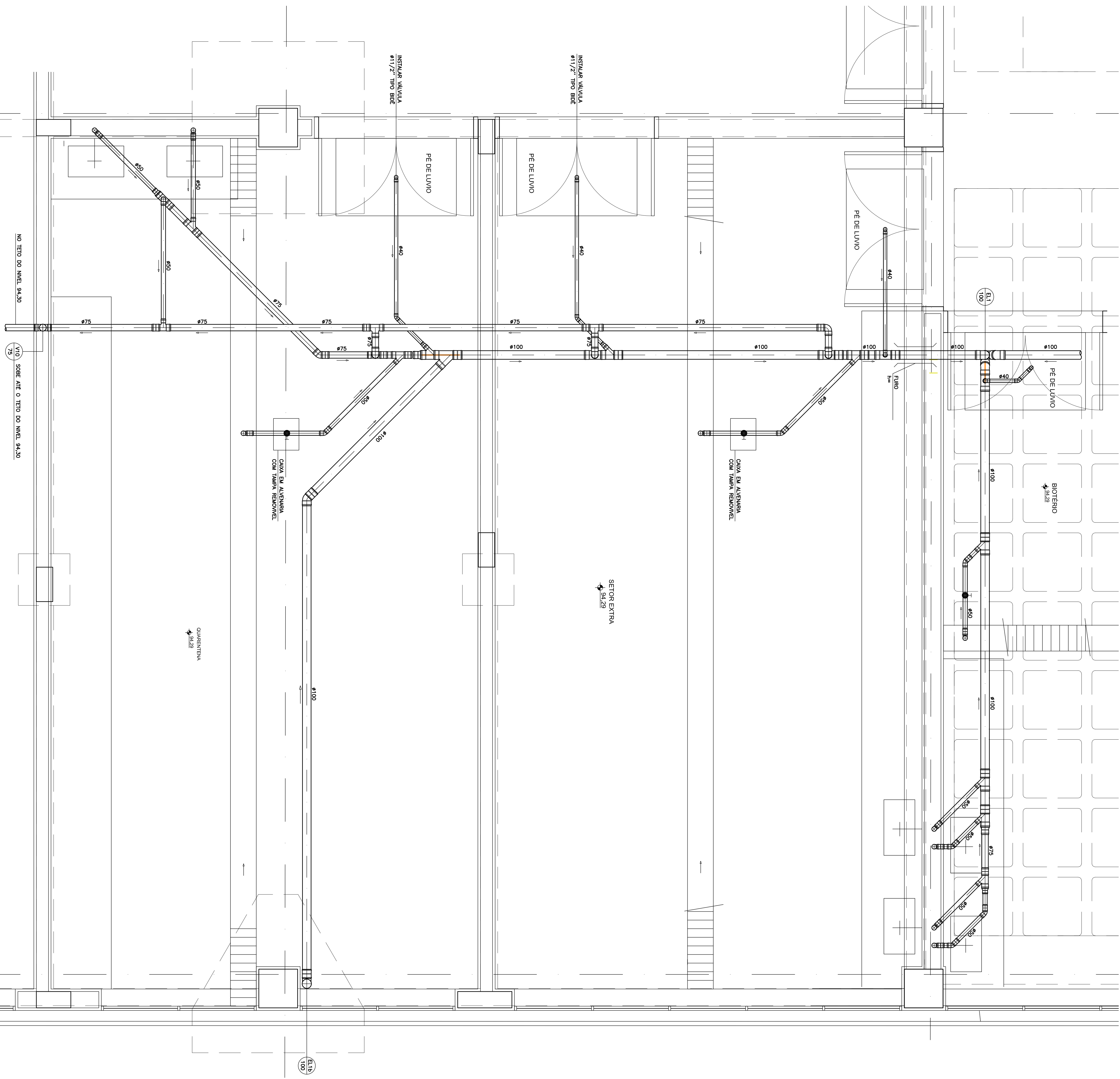
DETALHE ESCOTO - SETOR EXTRA
