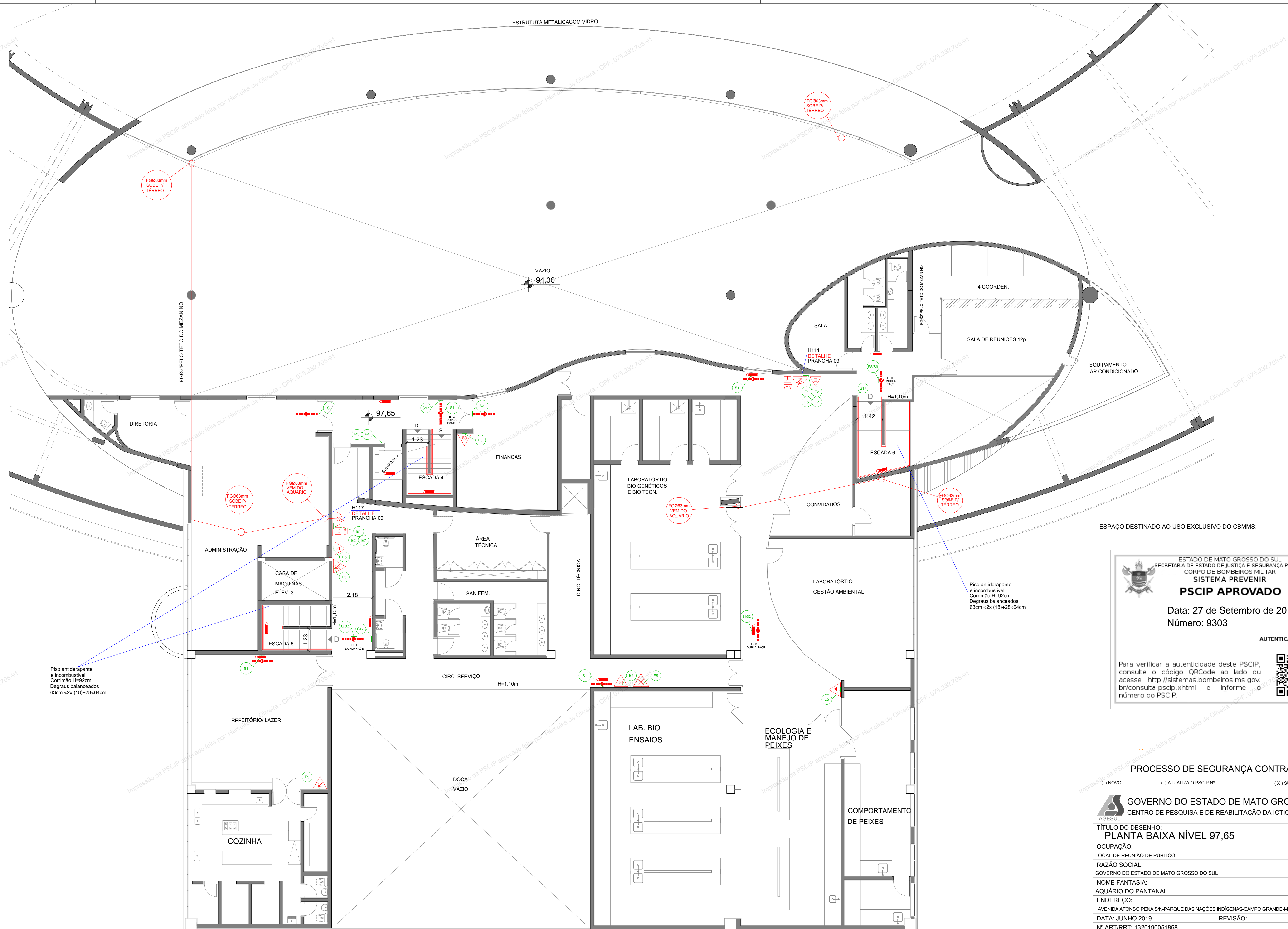
PLANTA BAIXA - NIVEL 97,65 ESCALA 1:100
