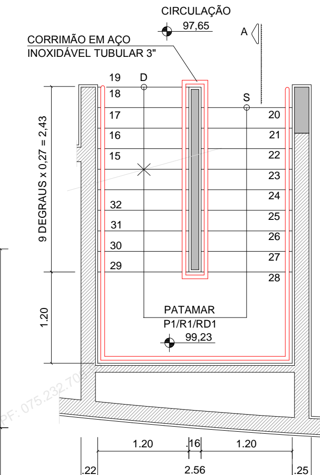
ESCADA 4 - PLANTA MEZANINO - NÍVEL 97,65 ESC.: 1:50
