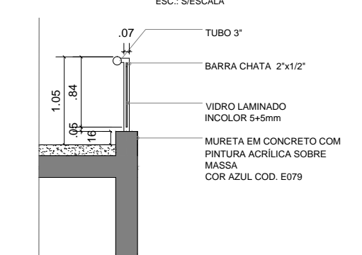
DET. ESCADA 4 ESC: S/ESCALA
