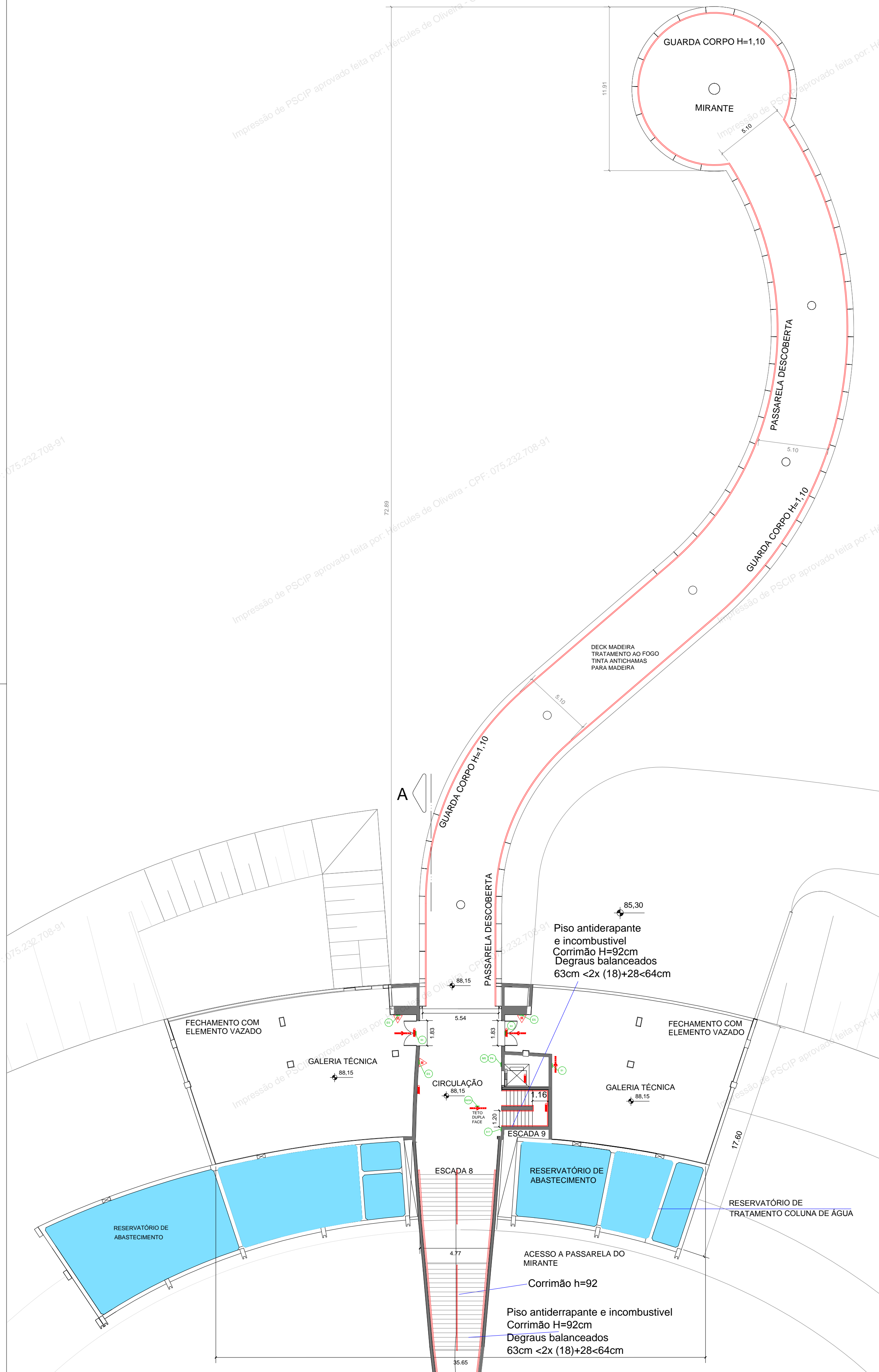
PAVIMENTO TÉCNICO SOB PASSARELA/MIRANTE-NÍVEL 85.35
