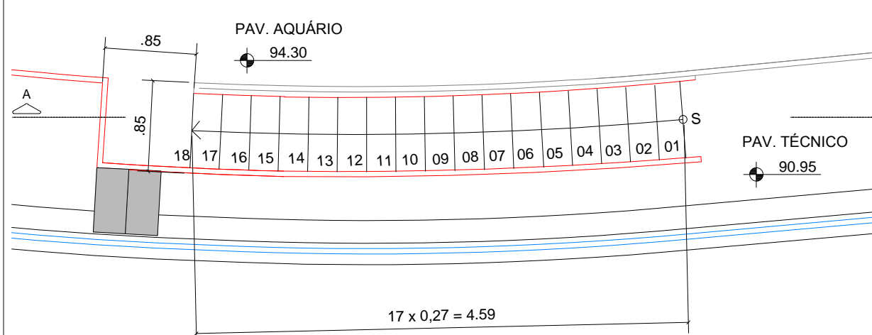
ESCADA TÉCNICA 10 - PLANTA PAV. AQUÁRIO - NÍVEL 94,30 ESC.: 1:50
