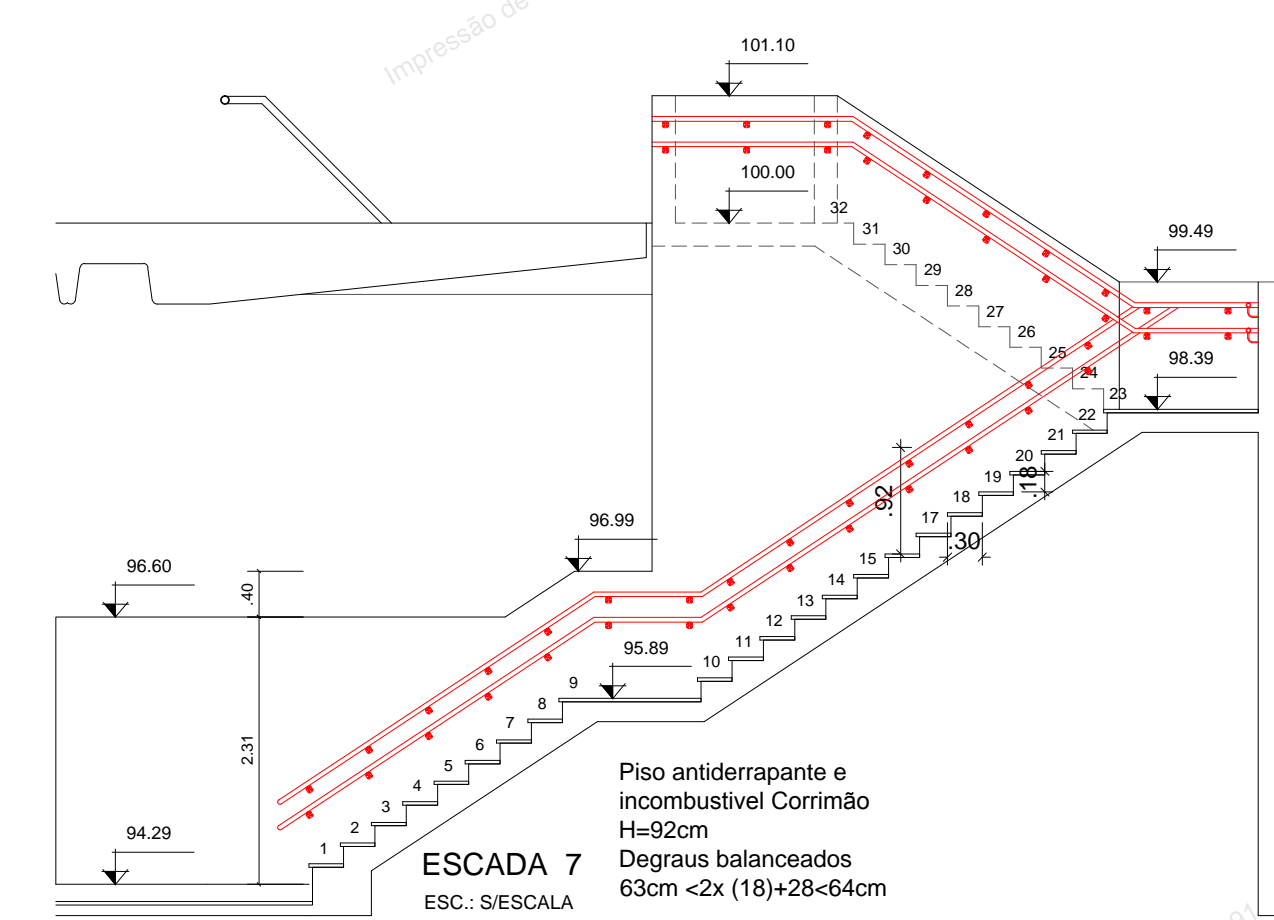
ESCADA 7 ESC: S/ESCALA
