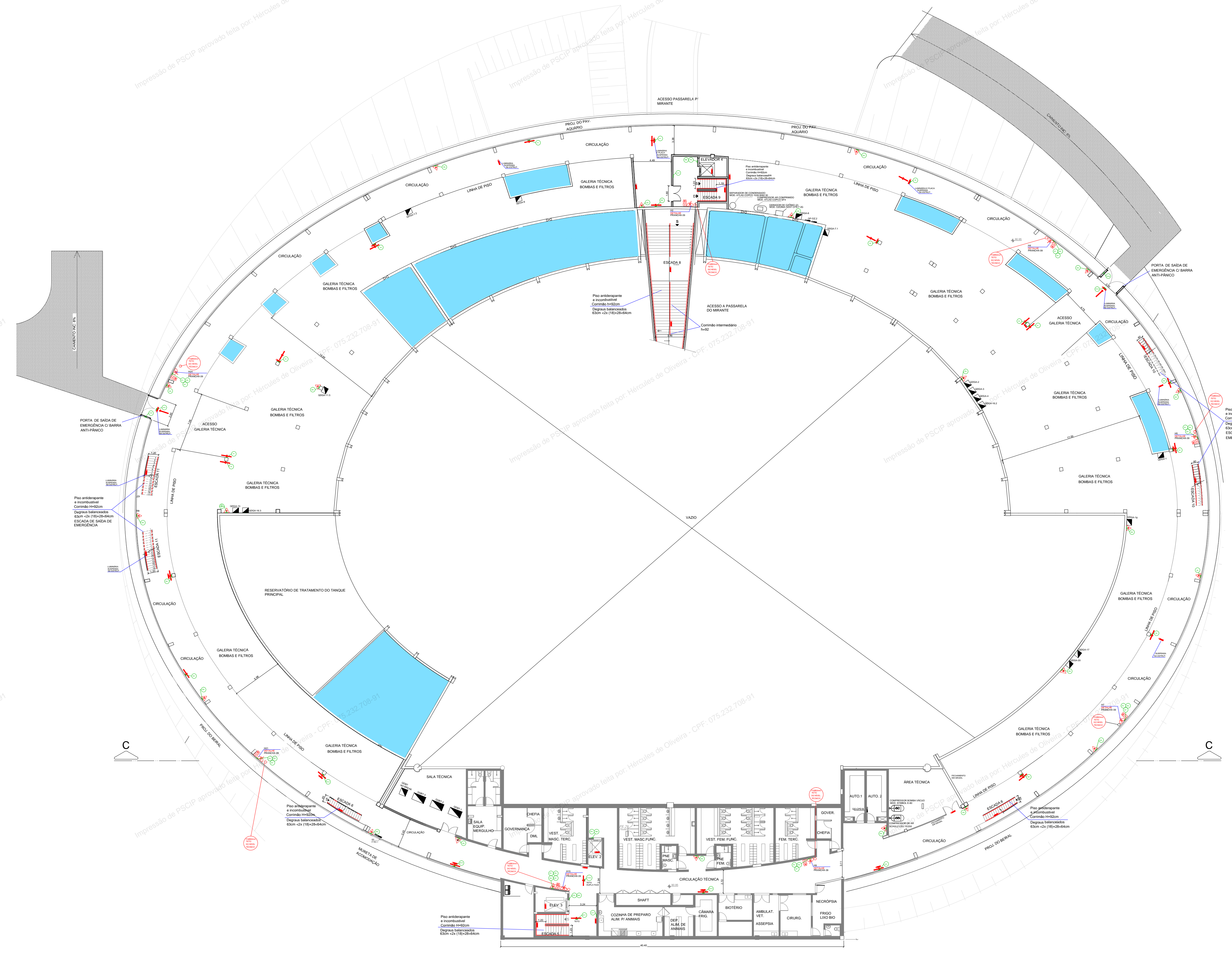
PAVIMENTO TÉCNICO SOB OS AQUÁRIOS-NÍVEL 90,95 ESC: 1/250
