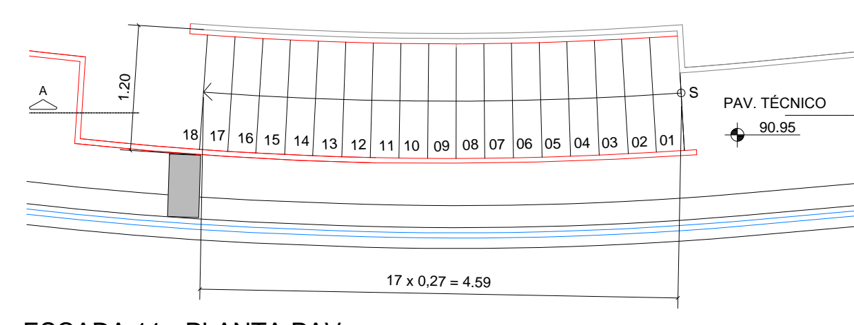
ESCADA 11 - PLANTA PAV. AQUÁRIO - NÍVEL 94,30 ESC.: 1:50
