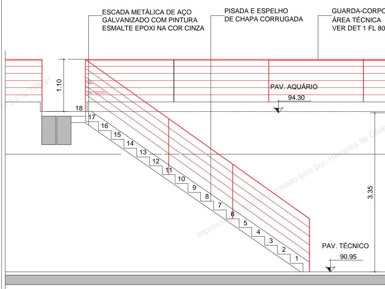
ESCADA 10 - SEÇÃO A ESC.: 1:50
