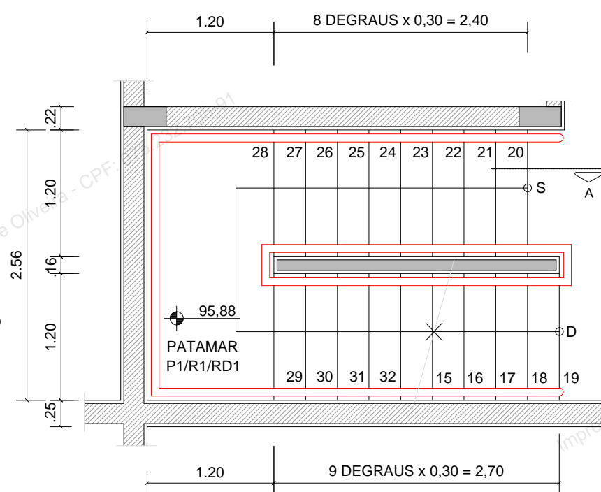
ESCADA 5 - PLANTA AQUÁRIO - NÍVEL 94,30 ESC.: 1:50
