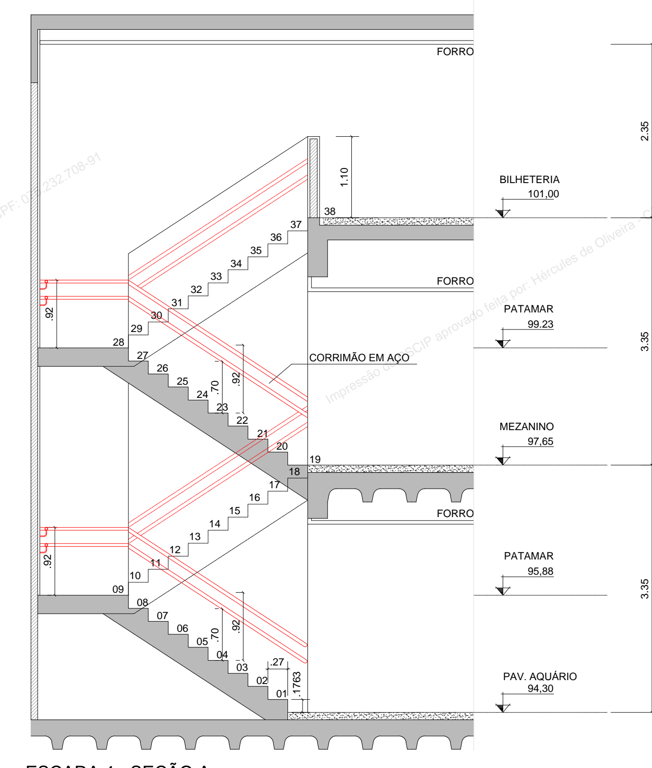
ESCADA 4 - SEÇÃO A ESC.: 1:50
