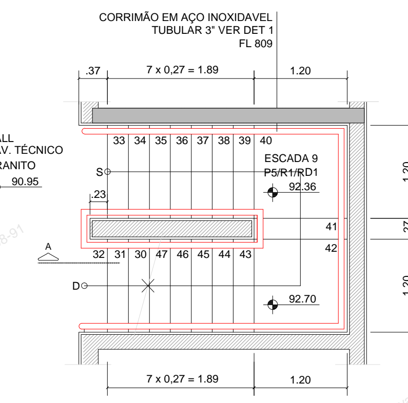
ESCADA 9 - PLANTA PAV. TÉCNICO - NÍVEL 90,95 ESC.: 1:50
