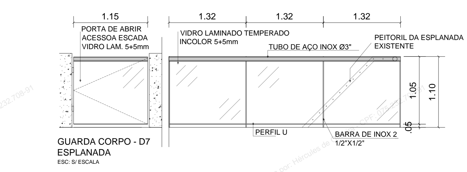
GUARDA CORPO - D7 ESPLANADA ESC: S/ESCALA
