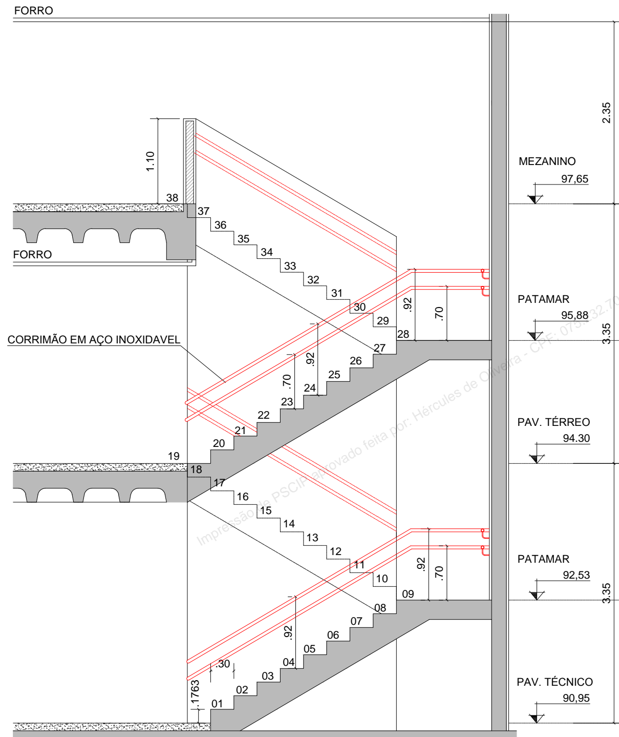
ESCADA 5 - SEÇÃO A ESC.: 1:50
