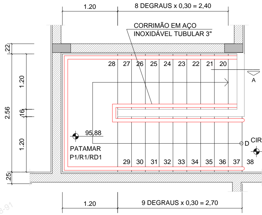
ESCADA 5 - PLANTA MEZANINO - NÍVEL 97,65 ESC.: 1:50
