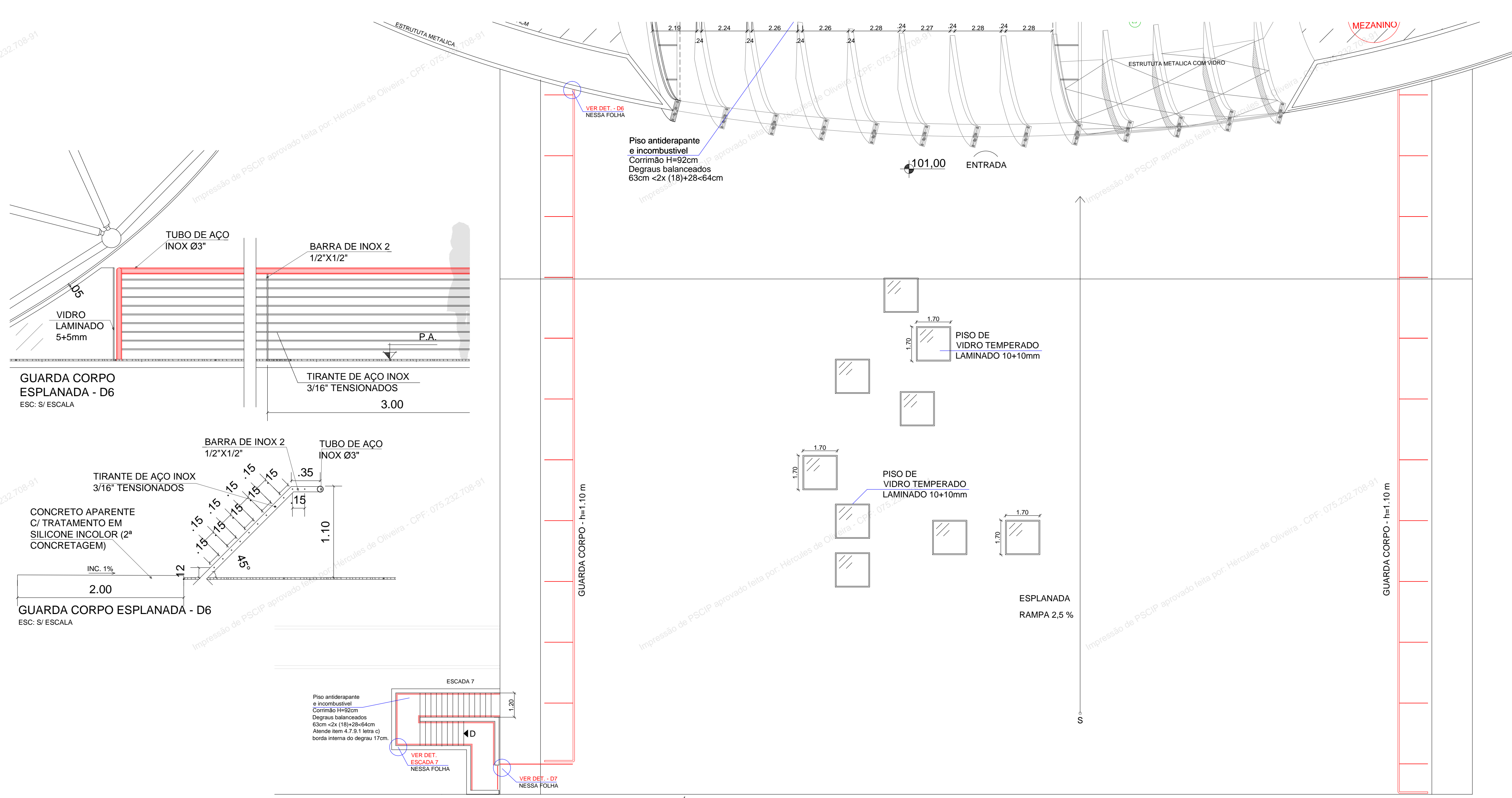
PLANTA BAIXA ESPLANADA TÉRREO ACESSO PRINCIPAL-NÍVEL 101.00 ESC: 1/125
