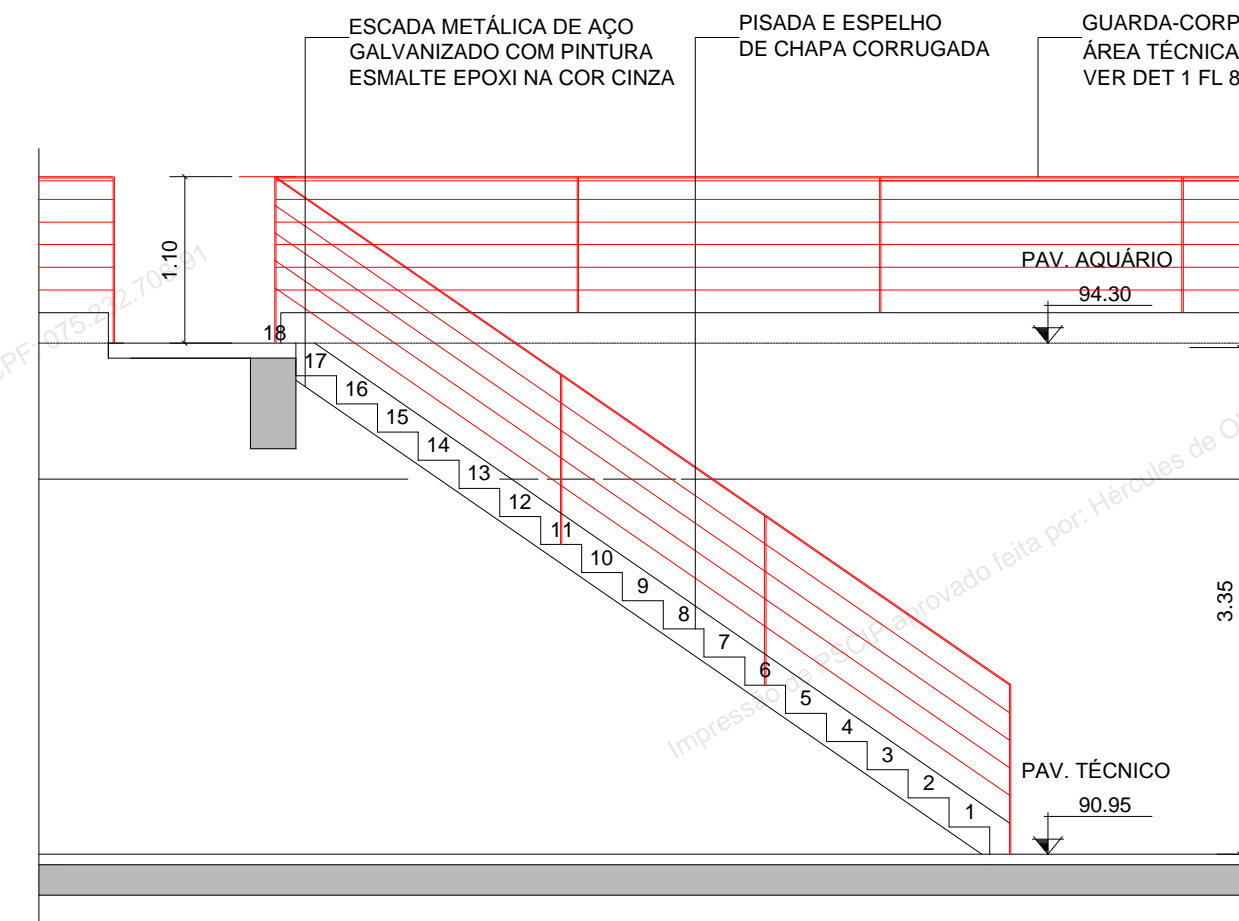
ESCADA 11 - SEÇÃO A ESC.: 1:50
