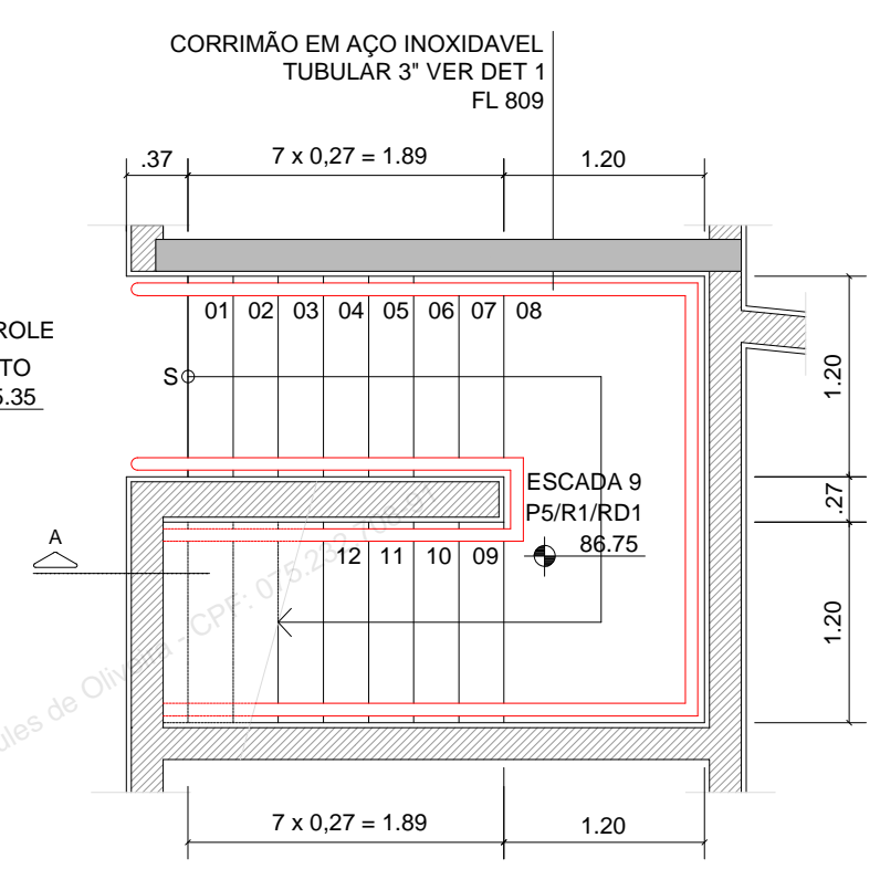
ESCADA 9 - PLANTA INFRAESTRUTURA - NÍVEL 85,35 ESC.: 1:50
