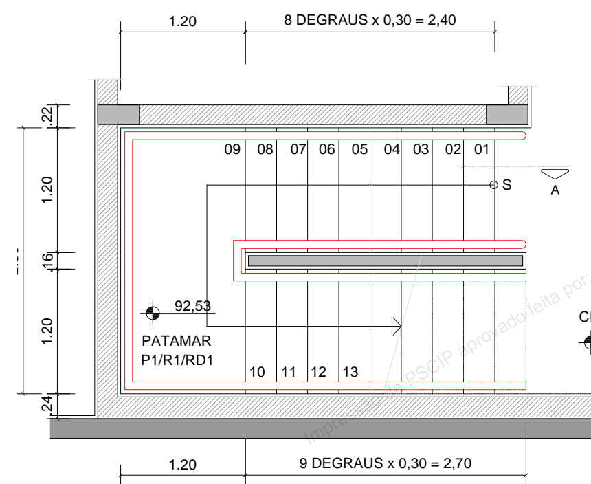
ESCADA 5 - PLANTA PAV. TÉCNICO - NÍVEL 90,95 ESC.: 1:50
