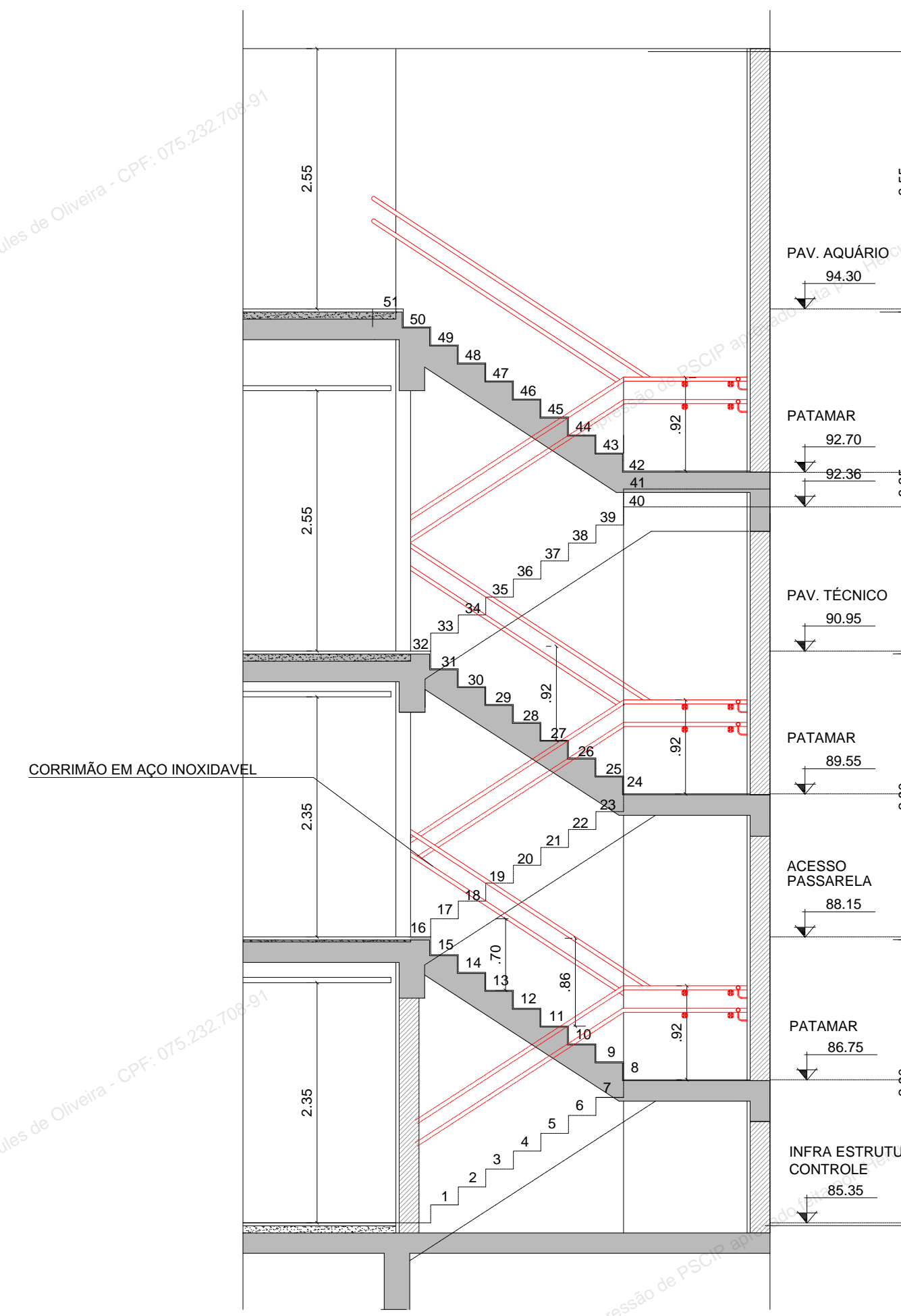
ESCADA 9 - SEÇÃO A ESC.: 1:50
