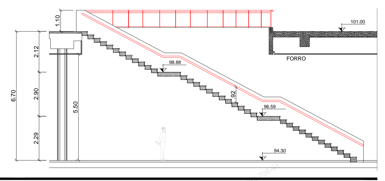
ESCADA 2 ESC: S/ESCALA
