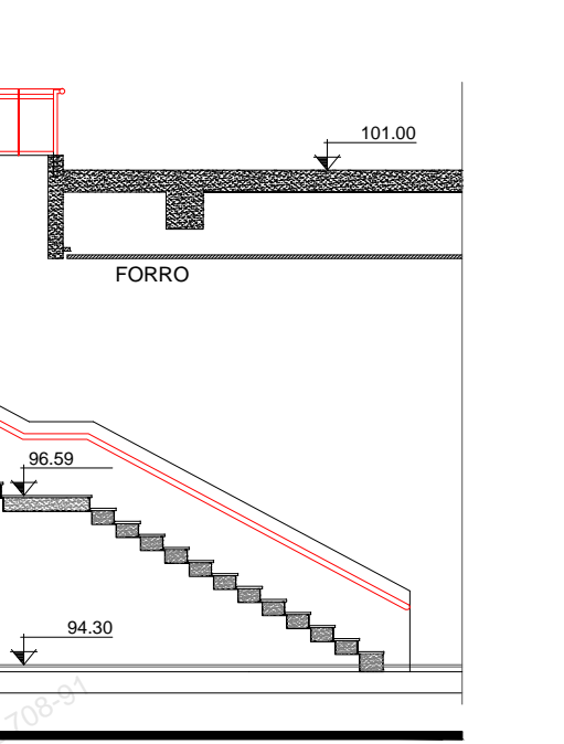
DET. ESCADA 2 ESC: S/ESCALA
