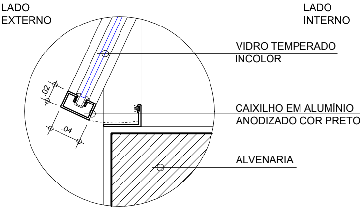
DET. 7 ESC.: 1:5
