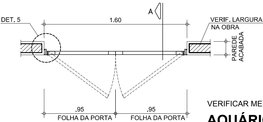
PLANTA - PV2 ESC. 1:25
