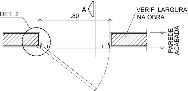
PLANTA - PF3 ESC. 1:25
