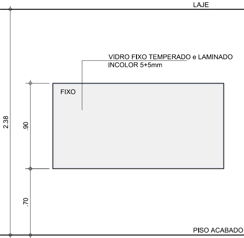
ELEVAÇÃO - VT14 ESC. 1:25
