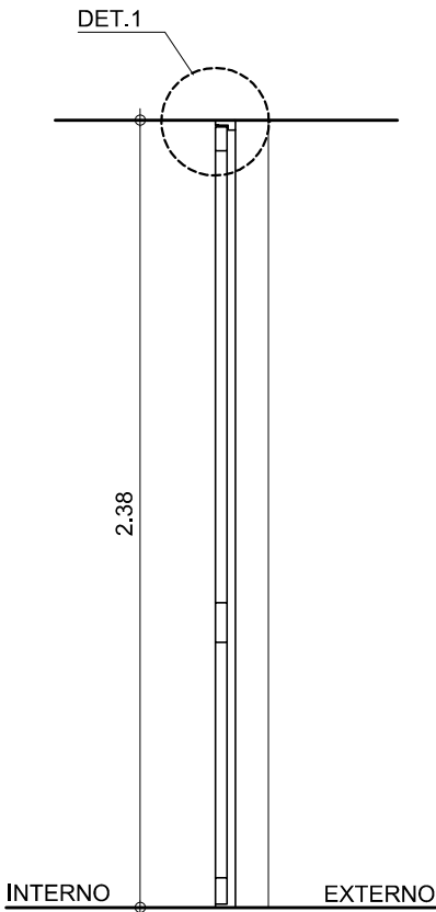
CORTE - PF2 ESC. 1:25
