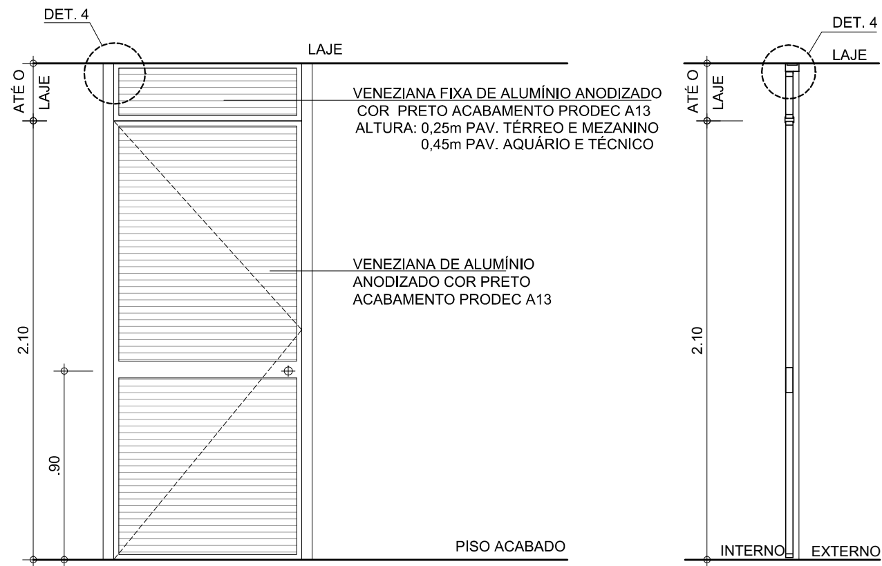
ELEVAÇÃO - PV1 ESC. 1:25
