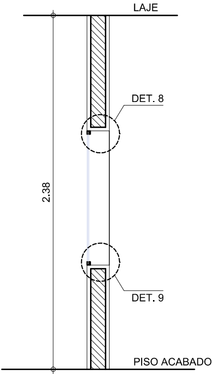
CORTE - VT14 ESC. 1:25
