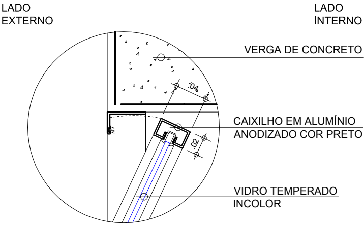
DET. 6 ESC.: 1:5
