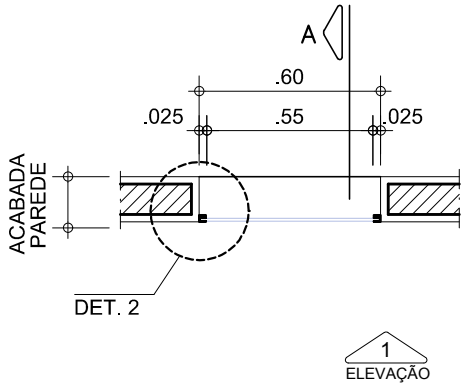
PLANTA - CF 21 ESC.: 1:25
