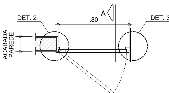
PLANTA - PF2 ESC. 1:25
