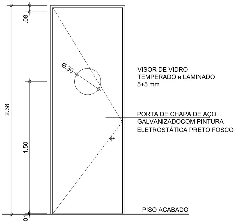
ELEVAÇÃO - PF2 ESC. 1:25
