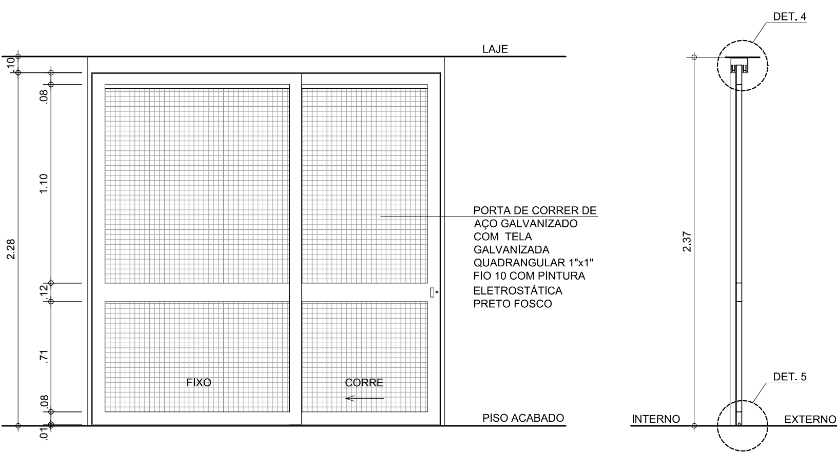
ELEVÇÃO - PF4 ESC. 1:25
