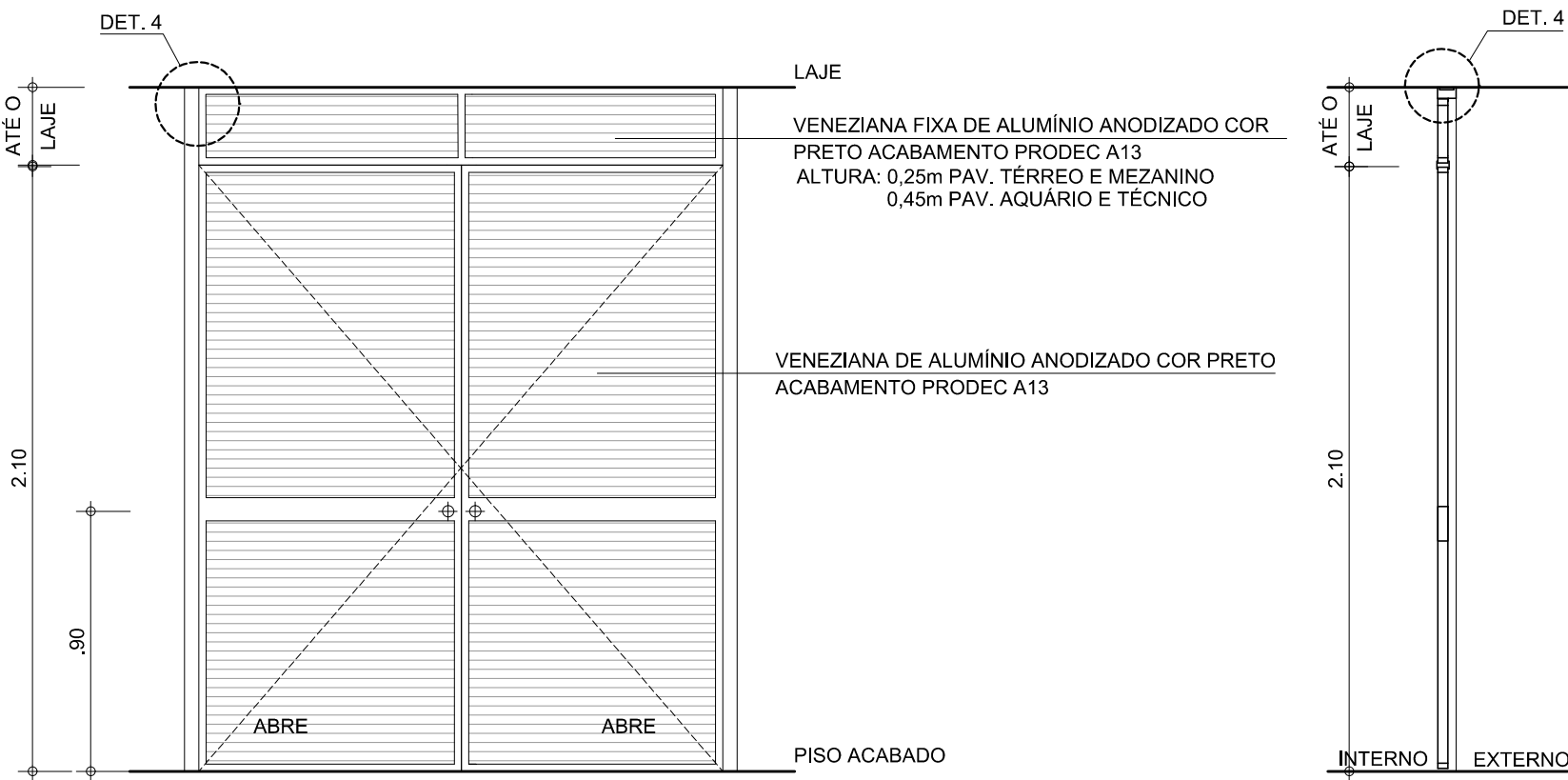
ELEVAÇÃO - PV2 ESC. 1:25
