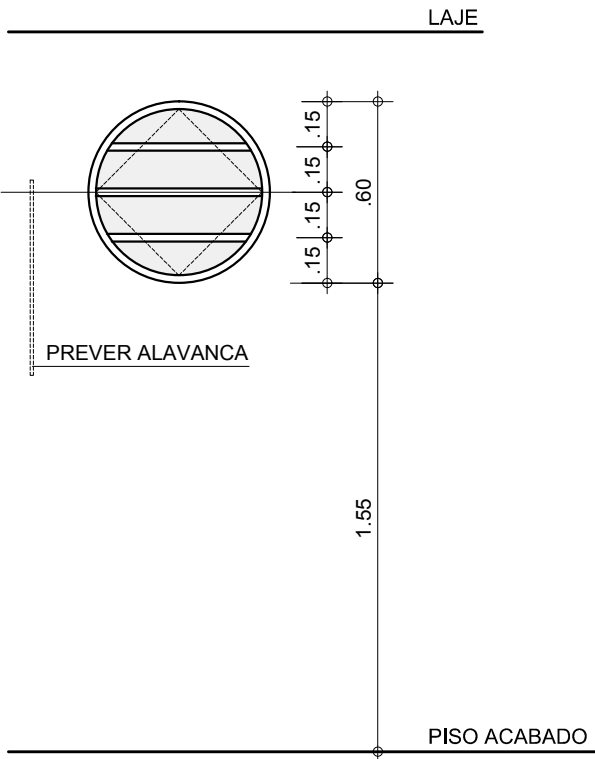
ELEVAÇÃO 1 - CF 21 ESC.: 1:25
