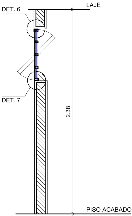
SEÇÃO A - CF 17 ESC.: 1:25
