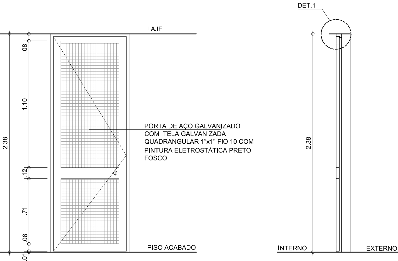
ELEVÇÃO - PF3 ESC. 1:25
