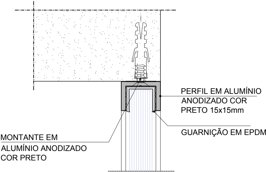
DET. 8 PLANTA ESC. 1:2
