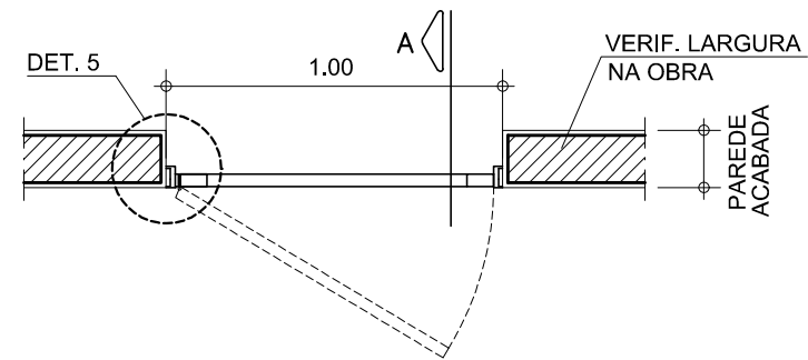
PLANTA - PV1 ESC. 1:25
