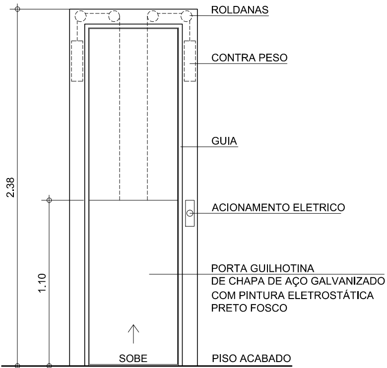
ELEVAÇÃO - PG1 ESC. 1:25
